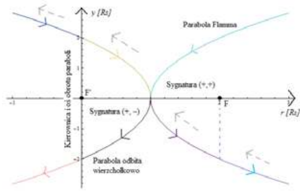
Rys. 1. Wykres paraboli Flamma oraz jej wierzchołkowego odbicia. Połowa ramion tych parabol jest zanurzona w zwykłej geometrii euklidesowej (górne albo nieodbite), a reszta w geometrii pseudoeuklidesowej (Minkowskiego, ramiona dolne albo odbite). Cały artykuł opiera się na tych parabolach. Rosnące fragmenty parabol dla r > 0 kodują metrykę Schwarzschilda na zewnątrz i wewnątrz horyzontu czarnej dziury. Fragmenty malejące parabol oraz fragment dla r < 0 są podstawą uogólnień do tzw. białych dziur kilku rodzajów. Zaznaczony jest zwrot ciążenia grawitacyjnego (w różnych przypadkach) oparty na analizie równań geodezyjnych wykonanej przez autora artykułu.
