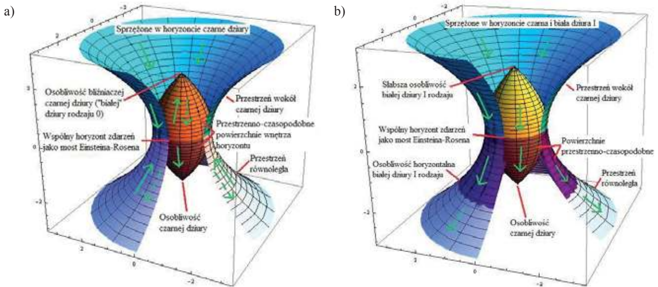
Rys. 3. Przedstawienie zanurzeniowe czarnej dziury „zsytej” z „białą” lub białą dziurą w horyzoncie zdarzeń będącym mostem Einsteina-Rosena z 1935 r. [4], jakościowo nawiązujące do rozszerzenia Kruskala-Szekeres z 1960 r. [15, 25], w przypadku: a) blizniaczej czarnej dziury – „białej” dziury rodzaju 0 (różna sygnatura dla r > R_S i r < R_S ), b) białej dziury I rodzaju (sygnatura zanurzenia określona znakiem y ). Zielone, ciągłe strzałki wskazują zwrot siły ciężarzenia wynikający z równań geodezyjnych, zaś strzałki przerywane mają zdaniem autora charakter spekulatywny.
