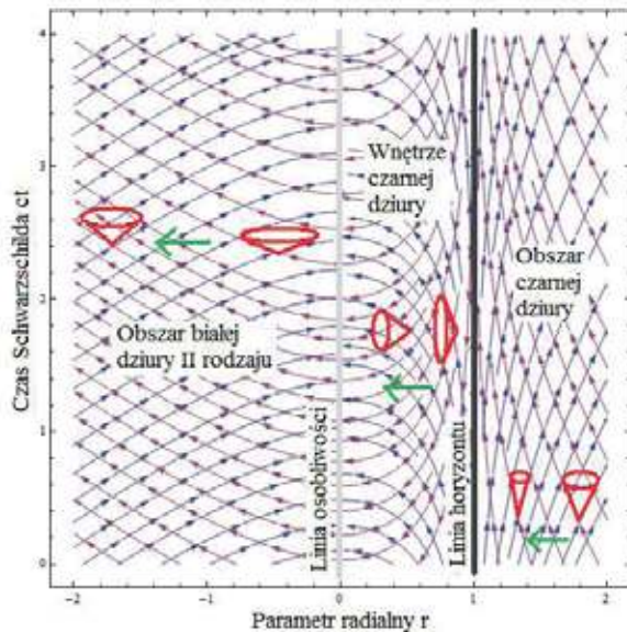
Rys. 7. Wykresy zorientowanych radialnych linii zerowych światła we współrzędnych Schwarzschilda dla: a) czarnej dziury i białej dziury II rodzaju, b) białej dziury I rodzaju i „białej” dziury III rodzaju. Zamykające się stożki świetlne przyszłości w tych współrzędnych wskazują zwrot ciążenia grawitacyjnego. Kryterium to potwierdzone we współrzędnych typu Schwarzschilda równaniami geodezyjnymi jest inspirowane podręcznikami [17, 26].
