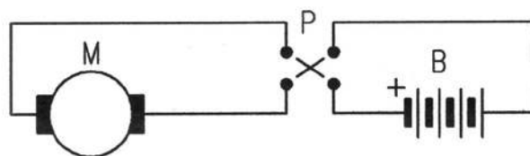
Rys. 7. Schemat obwodu mieszadełka: M – mikrosilnik na prąd stały, P – przełącznik, B – bateria.
