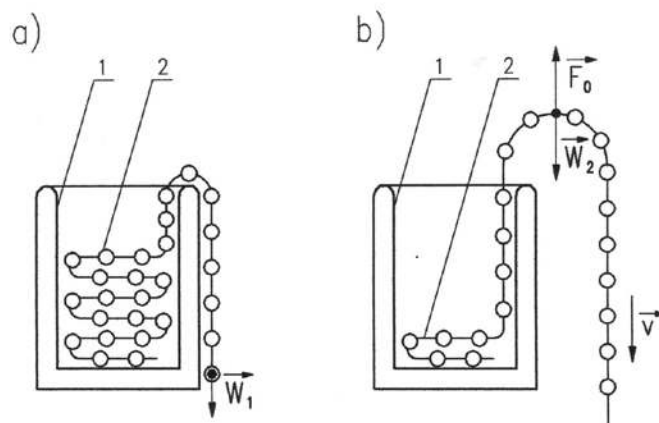
Rys. 6. Sposób przeprowadzenia doświadczenia z łańcuszkiem: a) sytuacja początkowa, b) sytuacja końcowa: 1 – małe naczynie szklane, 2 – łańcuszek, W_1 – ciężar wiszącej części łańcuszka, F_0 – siła odśrodkowa, W_2 – ciężar zewnętrznej części łańcuszka, v – prędkość łańcuszka.
