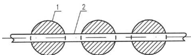
Rys. 5. Budowa łańcuszka pokazana w przekroju: 1 – kulka, 2 – linka.
