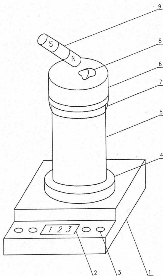
Rys. 1. Budowa układu doświadczalnego, 1 – waga jubilerska, 2 – wyświetlacz, 3 – przycisk włącznika, 4 – szalka, 5 – rurka, 6 – cienka folia polietylenowa, 7 – taśma klejąca, 8 – próbka badanej substancji, 9 – magnes neodymowy.
