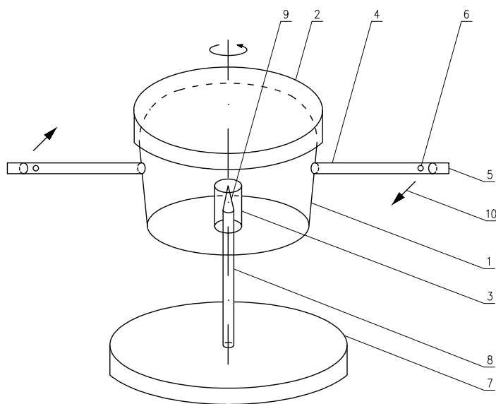
Rys. 1. Budowa modelu silnika odrzutowego; 1 – plastikowy przezroczysty pojemnik, 2 – zakrętka lub pokrywka pojemnika, 3 – probówka, 4 – słomka do napojów, 5 – zamknięty koniec słomki, 6 – otworek, 7 – podstawka, 8 – pręt, 9 – ostrze igły lub szpilki, 10 – strumienie dwutlenku węgla.
