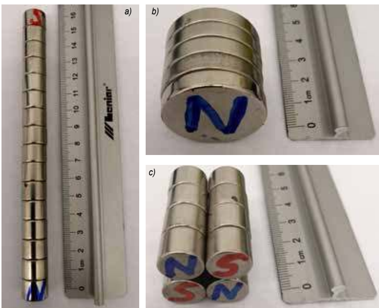
Fot. 2. Zestawy magnesów neodymowych używanych podczas doświadczeń: a) odpowiednik długiego magnesu sztabkowego, b) krótki magnes o zwiększonym polu przekroju poprzecznego, c) zestaw czterech krótkich magnesów o zwiększonym gradientie pola.
