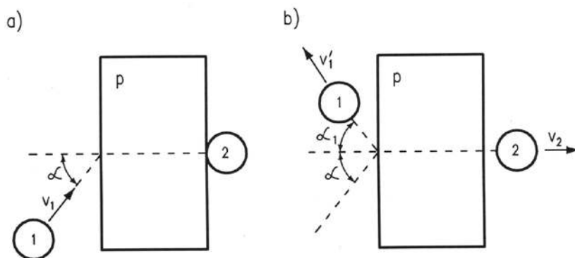
Rys. 7. Odbicie sprężyste skośne kulek od masywnej płytki prostokątnej: a) sytuacja przed odbiciem, b) sytuacja po odbiciu; p – płyta prostokątna o dużej masie, 1 – kulka nalicująca, 2 – kulka spoczywająca, \alpha , \alpha_1 – kąty odpowiednio: padania i odbicia kulki nalicującej, v_1 , v_1' , v_2 – prędkości odpowiednio: kulki nalicującej i kulki odbitej.
