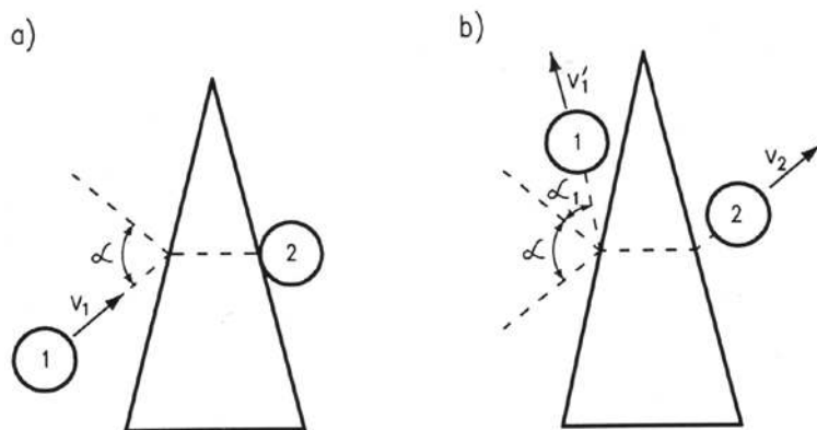
Rys. 8. Odbicie sprężyste skośne kulek od masywnej płytki w kształcie klina: a) sytuacja przed odbiciem, b) sytuacja po odbiciu; p – płyta w kształcie klina o dużej masie, 1 – kulka nalicująca, 2 – kulka spoczywająca, \alpha , \alpha_1 – kąty odpowiednio: padania i odbicia kulki nalicującej, v_1 , v_1' , v_2 – prędkości odpowiednio: kulki nalicującej i kulki odbitej.
