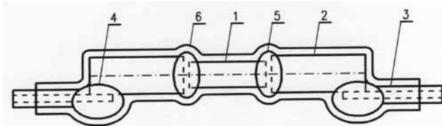
Rys. 3. Budowa hybrydowego elementu piezoelektrycznego, czulego również na pole magnetyczne; 1 – element piezoelektryczny, 2 – pręcik z materiału ferromagnetycznego, 3 – przewód, 4 – stop lutowiczny, 5 – klej przewodzący prąd elektryczny, 6 – rurka izolacyjna z folii termokurczliwej.
