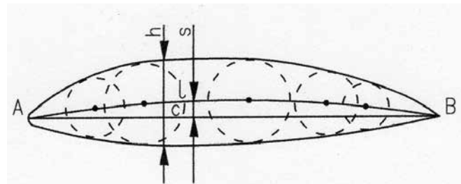
Rys. 1. Podstawowe elementy geometryczne profilu lotniczego, stanowiącego przekrój poprzeczny płata; A – nos, B – ogon, (nos i ogon są punktami przecięcia przekroju profilu przez krawędź natarcia i krawędź sypły), c – cięciwa, l – linia szkieletowa, s – strzałka, h – grubość.
