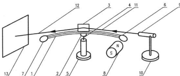
Rys. 1. Schemat układu doświadczalnego; 1 – cienka listewka sosnowa albo z balsy, 2 – końcówka wkładu do długopisu, 3 – zwierciadko płaskie z kawałka folii lustrzanej, 4 – cienka igła, 5 – podstawa igły, 6 – badany obiekt, np. owoc winogrona, 7 – przeciwcieżar, 8 – magnes trwały neodymowy, 9 – wskaźnik laserowy, 10 – podstawa wskaźnika laserowego, 11 – wiązka światła padająca, 12 – wiązka światła odbita, 13 – ekran.
