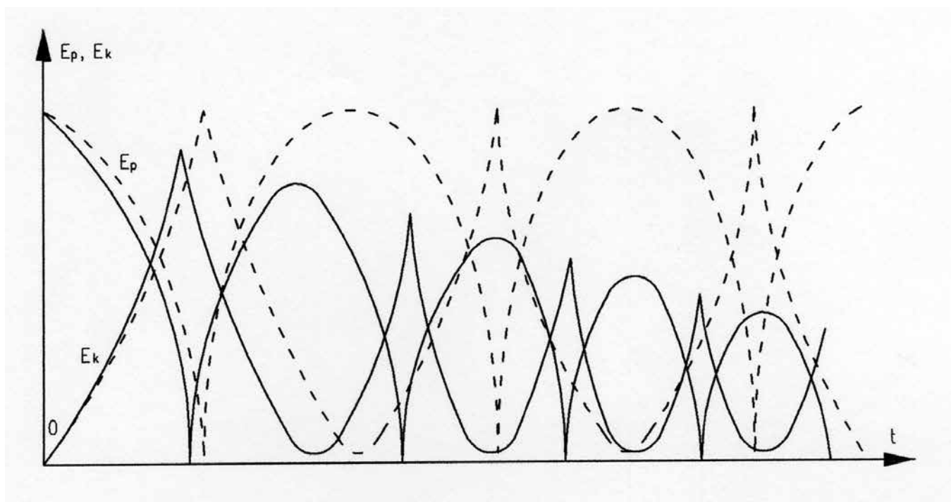
Rys. 7. Wykresy przedstawiające w sposób poglądowy zmiany energii potencjalnej E_p i energii kinetycznej E_k koła w kolejnych cyklach ruchu. Linie kreskowe odnoszą się do koła idealnego, poruszającego się bez oporów, natomiast linie ciągłe do koła rzeczywistego.
