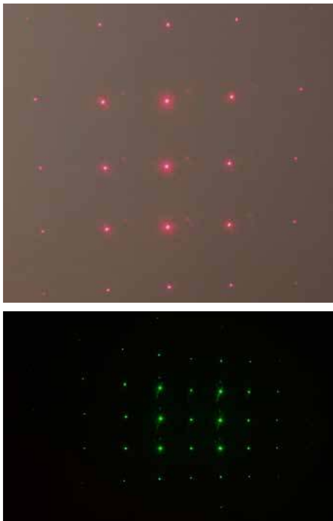
Fot. 3. Obrazy uzyskane na dwóch nałożonych na siebie siatkach dyfrakcyjnych 200 rys/mm przy wzajemnie prostopadłych kierunkach rys. Oświetlenie takie samo, jak w opisie fot. 2.
