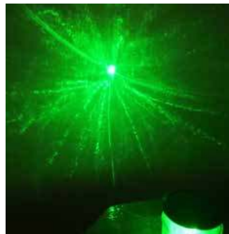
Fot. 6. Przykład obrazu otrzymanego w wyniku oświetlenia piany wiązką zielonego światła laserowego.
