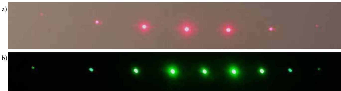
Fot. 2. Szeregi maksimów wytwarzane przez pojedyncze siatki dyfrakcyjne 200 rys/mm, oświetloną wskaźnikiem laserowym: a) czerwonym \lambda = 650 \text{ nm} , b) zielonym \lambda = 532 \text{ nm} .
