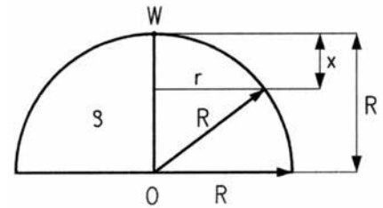
Rys. 4. Zależności geometryczne w przekroju pionowym przez oś półkolistego kopca, wykorzystywane do obliczenia zmiany natężenia pola grawitacyjnego na jego wierzchołku, \rho – gęstość materiału kopca.
