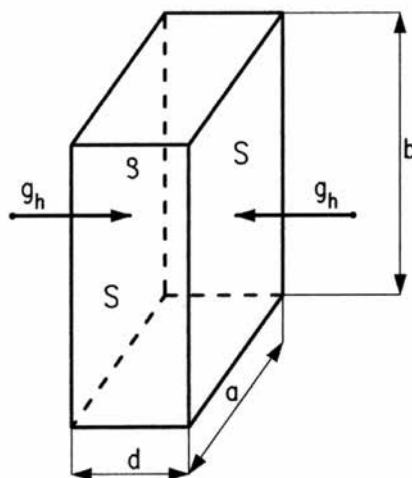
Rys. 2. Prostopadłościan wyodrębniony ze ściany w celu zastosowania prawa Gaussa dla pola grawitacyjnego; g_h – natężenie pola grawitacyjnego wytwarzane przez ścianę, S – powierzchnia użyta do obliczania strumienia natężenia, \rho – gęstość materiału skalnego ściany.
