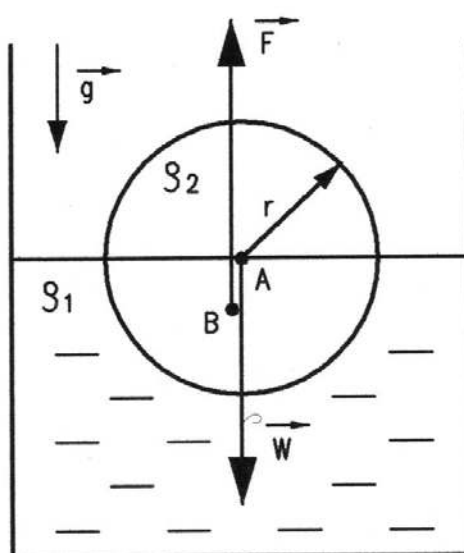
Rys. 3. Siły działające na pływającą kulę; W – ciężar kuli, F – siła wyporu, g – przyspieszenie ziemskie, \rho_1 – gęstość cieczy, \rho_2 – gęstość kuli, A – środek ciężkości kuli, B – środek wyporu (punkt przyłożenia siły wyporu), r – promień kuli.
