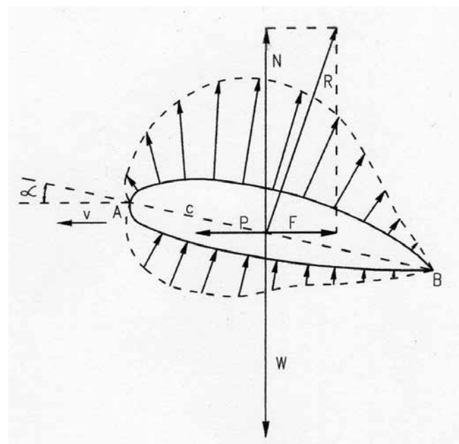
Rys. 3. Rozkład ciśnienia wokół płata i siły działające na płat w locie ustalonym; \mathbf{R} – wypadkowa siła aerodynamiczna, \mathbf{N} – siła nośna, \mathbf{F} – siła oporu aerodynamicznego, \mathbf{P} – siła napędu, \mathbf{W} – ciężar, v – prędkość lotu, \alpha – kąt natarcia, A – nos, B – ostrze, c – cięciwa.
