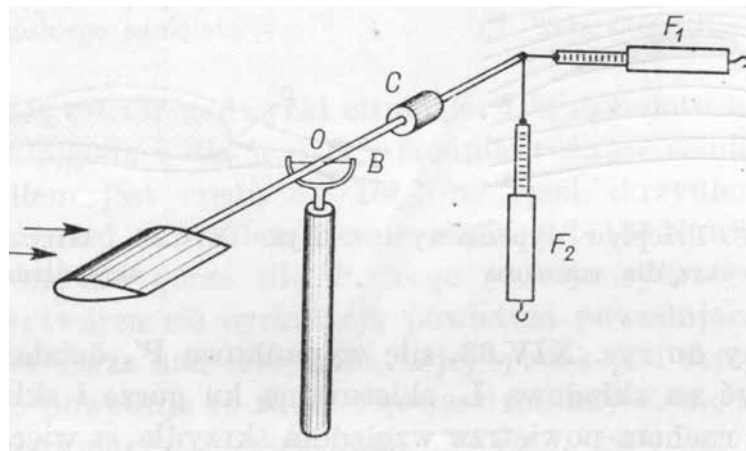
Rys. 5. Schemat wagi aerodynamicznej; O – oś pionowa, B – oś pozioma, C – ciężarek, F_1, F_2 – siłomierze do pomiaru siły oporu i siły nośnej, źródło [2].
