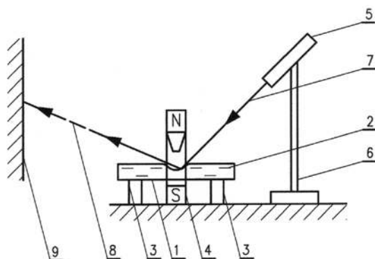
Rys. 4. Schemat układu do obserwacji efektu Mojżesza za pomocą wiązki światła laserowego; 1 – otwarte przezroczyste naczynie z poczerzonym dnem, 2 – ciecz diamagnetyczna, 3 – wspornik, 4 – magnes neodymowy z nabiegunnikiem, 5 – wskaźnik laserowy, 6 – statyw, 7, 8 – wiązka światła odpowiednio: padająca i odbita, 9 – ekran.
