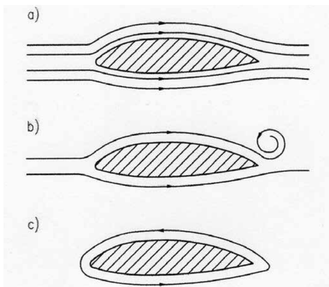
Rys. 2. Różne warianty opływu płata: a) laminarny, b) z wirami rozruchowymi za krawędzią spływu, c) z wirami wokół płata.
