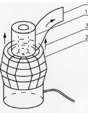
Rys. 4. Inny wariant układu do badania siły nośnej; 1 – rolka papieru toaletowego, 2 – osłona śmigła wentylatora, 3 – strumień powietrza, 4 – unoszony fragment papieru toaletowego.
