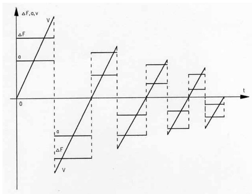
Rys. 6. Wykresy przedstawiające w sposób poglądowy zmiany siły naprężenia nici \Delta F , przyspieszenia liniowego a oraz prędkości liniowej v w czterech początkowych cyklach ruchu koła.
