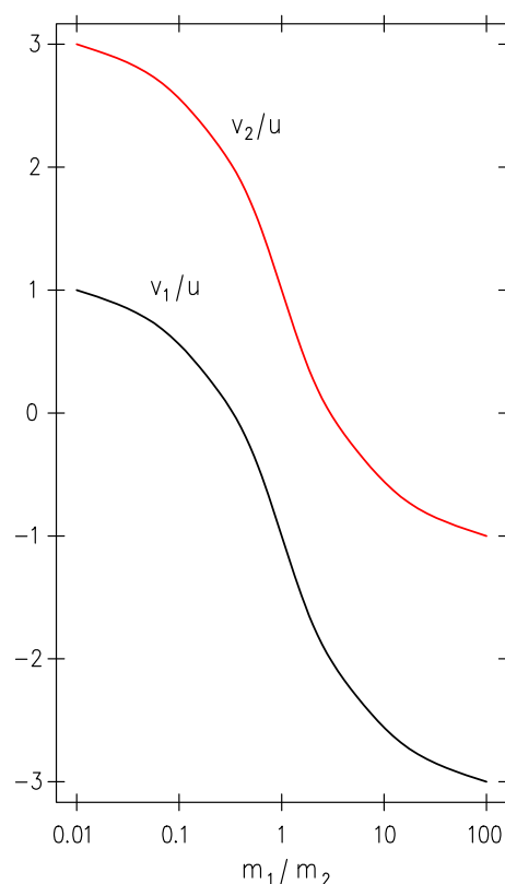
prędkości kulek po zderzeniu sprężystym v_1/u , v_2/u w zależności od ich stosunku mas m_1/m_2 wyrażonego w skali logarymicznej.
