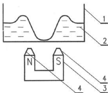
Rys. 3. Sposób wytworzenia prostego efektu Mojżesza w cieczy paramagnetycznej; 1 – otwarte przezroczyste naczynie, 2 – ciecz paramagnetyczna, 3 – magnes neodymowy, 4 – nabiegunnik.
