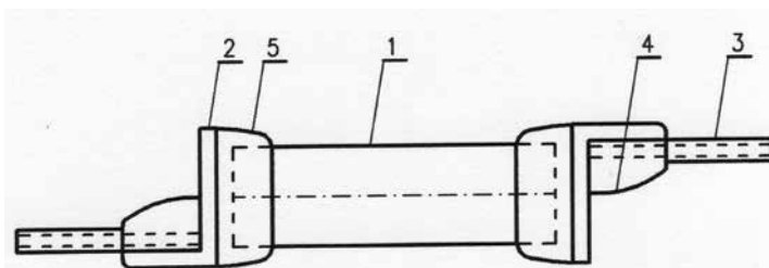
Rys. 1. Najprostszy sposób przyłączenia elektrod do kryształu piezoelektrycznego; 1 – element piezoelektryczny, 2 – elektrody z pasków blachy miedzianej albo mosiężnej, 3 – przewody, 4 – stop lutowniczy, 5 – klej przewodzący prąd elektryczny.
