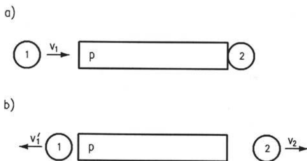
Rys. 3. Zderzenie sprężyste z masywną płytą dwóch kulek, spadających razem: a) sytuacja przed zderzeniem, b) sytuacja po zderzeniu; 1, 2 – kulki odpowiednio: o mniejszej i o większej masie, h_1 , h_2 – maksymalne wzniesienia środków masy nad płytą odpowiednio: układu obu kulek, kulki o mniejszej masie i kulki o większej masie.
