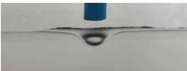
Fot. 4. Efekt Mojżesza spowodowany przez strumień powietrza, wypływający z rurki prostopadle na powierzchnię wody.
