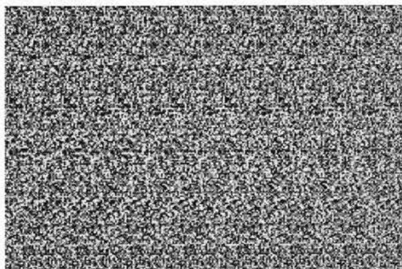
Rys. 5. Przykłady stereogramów utworzonych z pojedynczych, przypadkowo rozmieszczonych punktów. Przy odpowiednim sposobie patrzenia na rys. a) pojawia się przestrzenna spirala, a na rys. b) układ kulek umieszczonych w rzędach.
