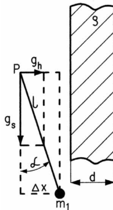
Rys. 1. Odchylenie kulki zawieszonoj na nici w pobliżu masywnej ściany skalnej; g_s – średnie przyspieszenie ziemskie, g_h – natężenie pola grawitacyjnego, wytwarzane przez ścianę, l – długość nici, m_1 – masa kulki, \rho – gęstość materiału skalnego ściany.
