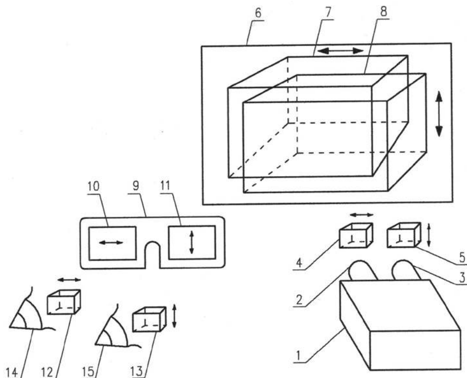
Rys. 3. Wyjaśnienie wizualizacji przestrzennej przy użyciu światła spolaryzowanego; 1 – projektor, 2 – lewy obiektyw, 3 – prawy obiektyw, 4 – obraz prostopadłością widzianego przez lewe oko w świetle spolaryzowanym poziomo, 5 – obraz prostopadłością widzianego przez prawe oko w świetle spolaryzowanym pionowo, 6 – ekran, 7 – rzut prostopadłością z lewego obiektywu, 8 – rzut prostopadłością z prawego obiektywu, 9 – oprawka okularów, 10 – polaryzator mający kierunek polaryzacji skierowany poziomo, 11 – polaryzator mający kierunek polaryzacji skierowany pionowo, 12 – obraz sześcianu w świetle spolaryzowanym poziomo, 13 – obraz sześcianu w świetle spolaryzowanym pionowo, 14 – lewe oko, 15 – prawe oko.
