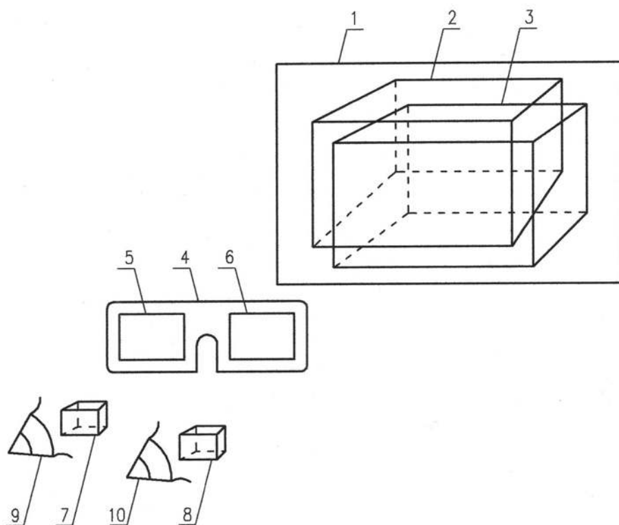
Rys. 2. Wyjaśnienie wizualizacji przestrzennej przy użyciu anaglifów; 1 – tablica, 2 – rzut prostopadłością widzianego przez lewe oko w kolorze niebieskim, 3 – rzut prostopadłością widzianego przez prawe oko w kolorze czerwonym, 4 – oprawka okularów, 5 – filtr optyczny niebieski, 6 – filtr optyczny czerwony, 7 – obraz sześcianu w kolorze niebieskim, 8 – obraz sześcianu w kolorze czerwonym, 9 – lewe oko, 10 – prawe oko.
