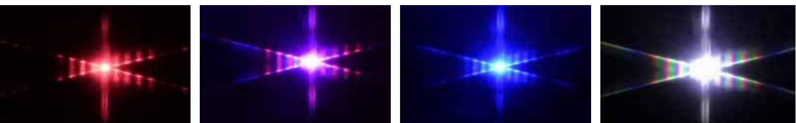
Fot. 7. Obrazy wytworzone z wyniku dyfrakcji na ekranie tego samego odbiornika telewizyjnego z matrycą ciekłokrystaliczną, oświetlonego wskaźnikiem laserowym w kolorze: a) czerwonym \lambda = 650 \text{ nm} , b) zielonym \lambda = 532 \text{ nm} , c) niebieskim \lambda = 450 \text{ nm} , a ponadto d) oświetlonego światłem białym, emitowanym przez OLED (organiczną diodę elektroluminescencyjną) z latarki czołowej.
