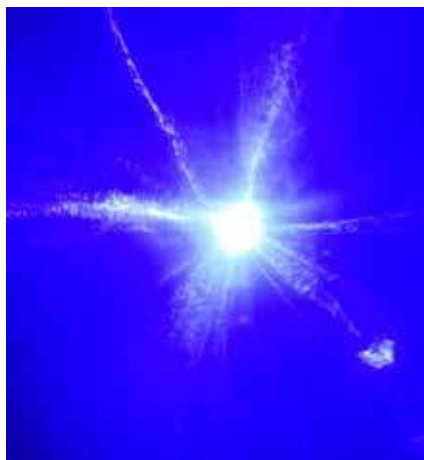
Fot. 4. Przykład obrazu otrzymanego w wyniku oświetlenia piany wiązką niebieskiego światła laserowego.
