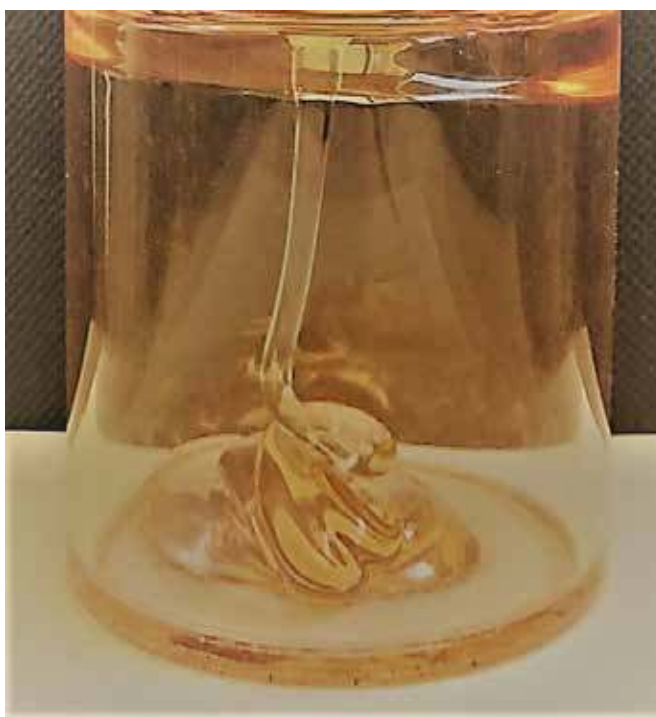
Fot. 6 Odskok hydrauliczny i rozptyw cieczy nienewtonowskiej o bardzo dużej lepkości w tzw. klepsydze żelowej (efekt Fano).
