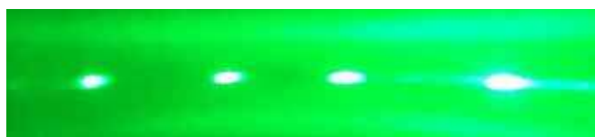
Fot. 4. Szereg maksimów wytworzonych na płycie DVD oświetlonej czerwonym wskaźnikiem laserowym \lambda = 650 \text{ nm} .
