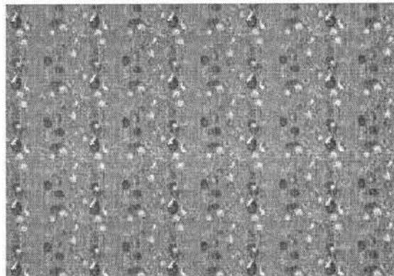
Rys. 5. Przykłady stereogramów utworzonych z pojedynczych, przypadkowo rozmieszczonych punktów. Przy odpowiednim sposobie patrzenia na rys. a) pojawia się przestrzenna spirala, a na rys. b) układ kulek umieszczonych w rzędach.
