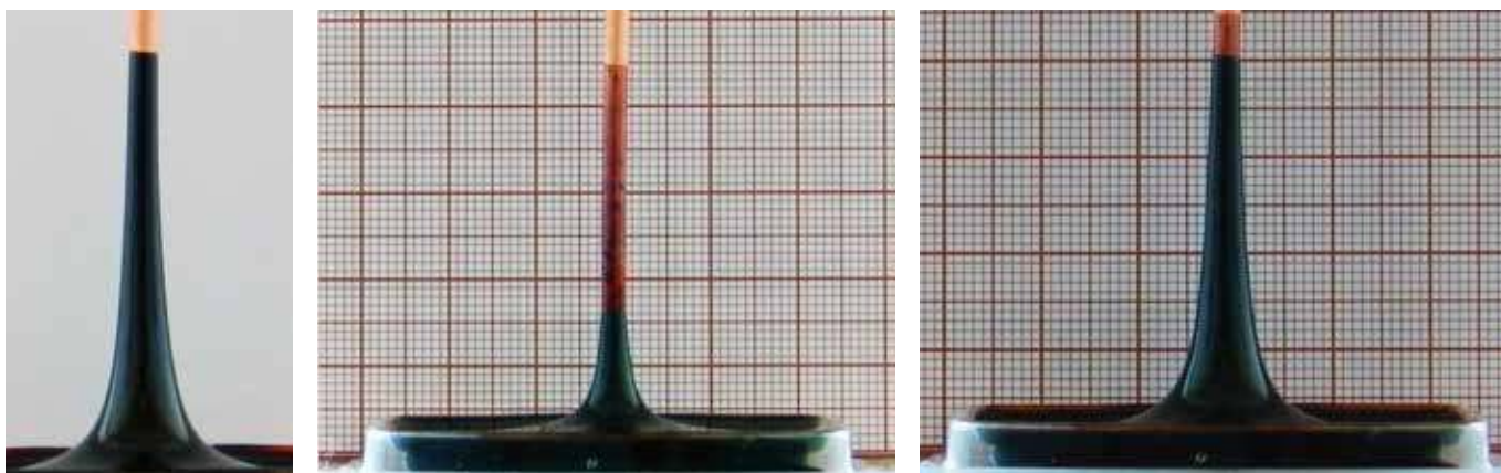
Fot. 2. Efekt Moirésa w polu magnetycznym, wytwarzanym przez prąd elektryczny, przepływający w prostoliniowym odcinku drutu – kolumny ferrofluidu otrzymane podczas wzrostu natężenia prądu.
