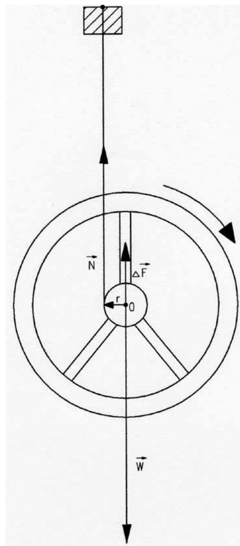
Rys. 4. Siły działające w układzie koła podczas ruchu w dół; W – ciężar koła, N – suma sił naprężenia nici, \Delta F – siła bezwładności (zmiana ciężaru koła), r – promień koła, O – środek osi.
