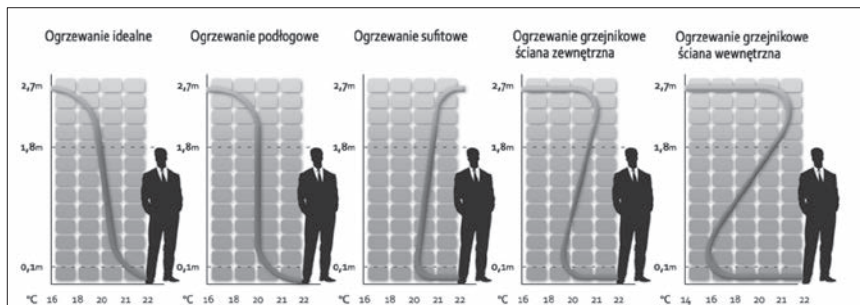
Rys. 3. Wykres przedstawiający różnicę rozkładu temperatur w przypadku różnych systemów ogrzewania Źródło: Thermo-Vitae
