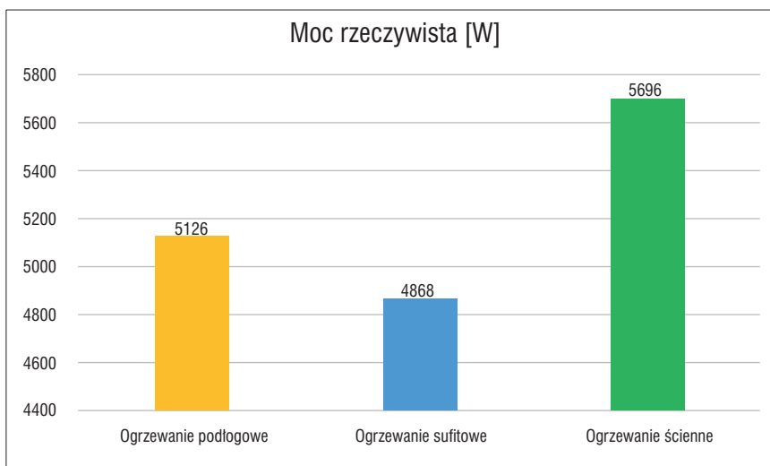
Rys. 2. Zestawienie wyników rzeczywistych mocy grzewczych porównywanych systemów ogrzewania płaszczyznowego Źródło: obliczenia własne
