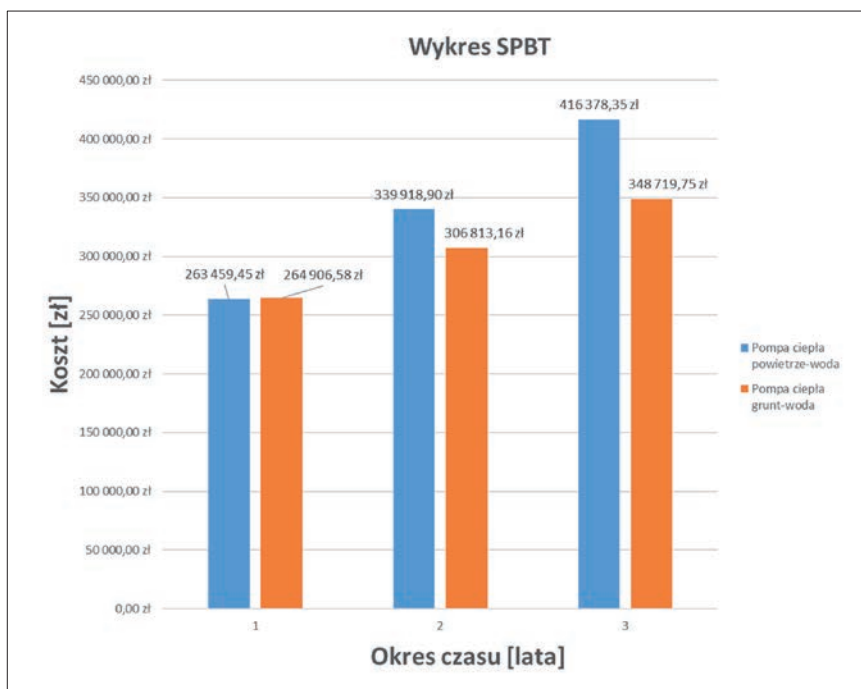
Rys. 3. SPBT – prosty okres zwrotu. Porównanie obu wariantów inwestycji pod względem kosztów początkowych i kosztów eksploatacyjnych w kolejnych latach pracy instalacji
