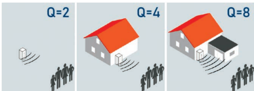
Rys. 1. Ustawienie pompy ciepła a współczynnik kierunkowości Q
