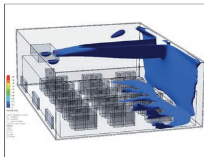
Fot. 2. Izopowierzchnia demonstrująca przestrzeń o prędkości powietrza 0,5 m/s lub wyższej
