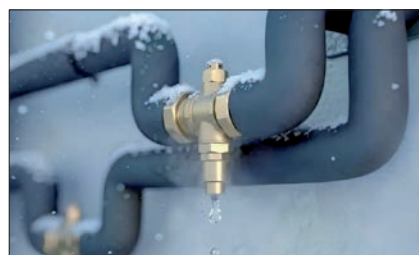
Fot. 5. Zawór antyzamrozeniowy
