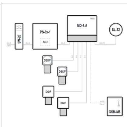
Rys. 1. Progowy system detekcji gazów dla mniejszych oczyszczalni
