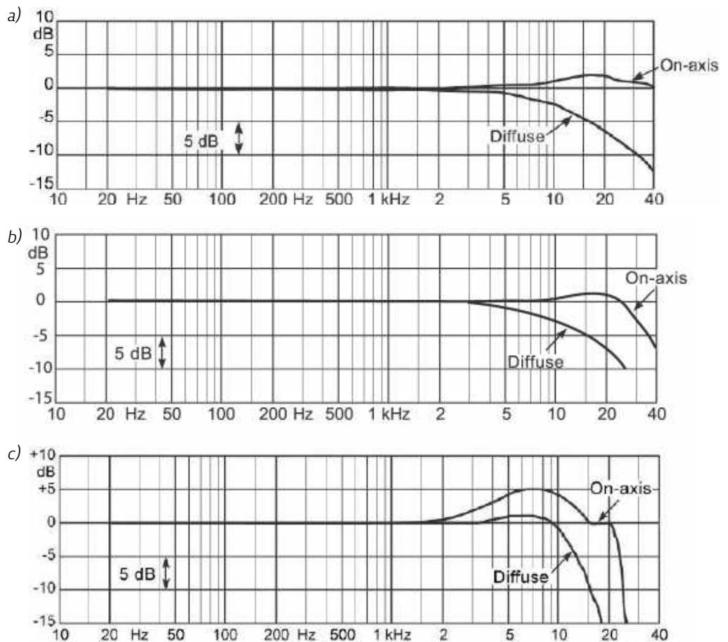
Rysunek 1. Częstotliwościowe charakterystyki amplitudowe ilustrujące szerokość pasma przenoszenia mikrofonów z membraną o średnicy: a) 12 mm, b) 16 mm, c) 24 mm.
