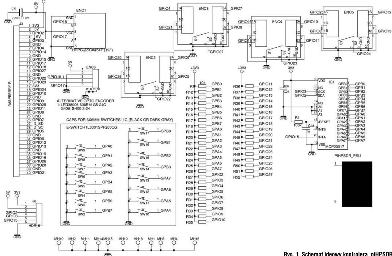
Rys. 1. Schemat ideowy kontrolera piHPSDR
