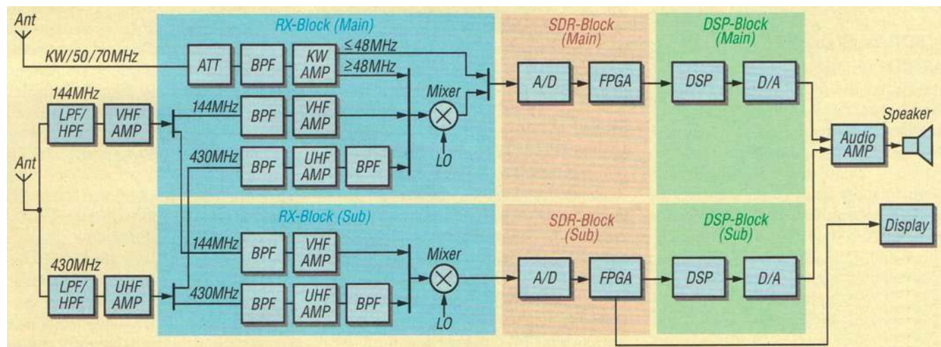
Rys. 7. Schemat blokowy transceivera Yaesu FTX-1 Field
