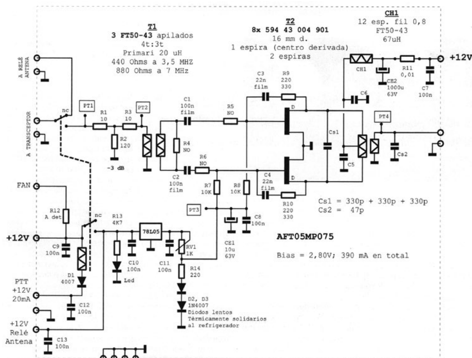
Rys. 5. Schemat ideowy liniowego y wzmacniacz mocy HF
