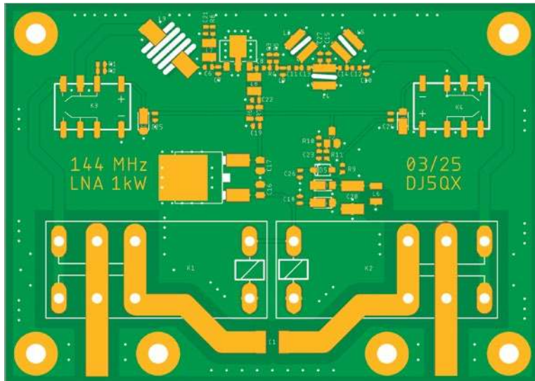
Rys. 2. Schemat montażu płytki przedwzmacniacza 2 m, oryginalne wymiary: 70 mm x 50 mm
