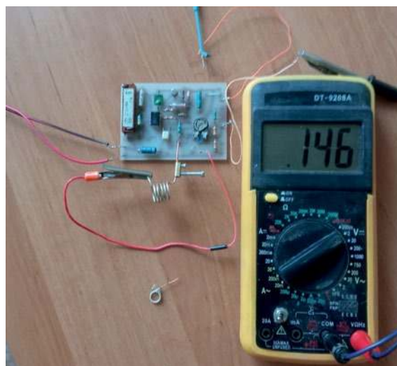
Napięcia przy pomiarach różnych cewek
