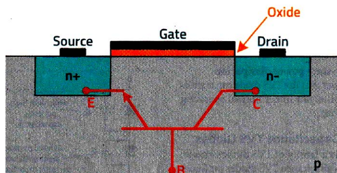
Rysunek 5. Pasożytniczy tranzystor bipolarny w strukturze tranzystora NMOS. Emiterem jest źródło, kolektorem dren, a bazą podłoża typu p pod kanałem. Źródło: H. Zenkner, Würth Elektronik eiSos
