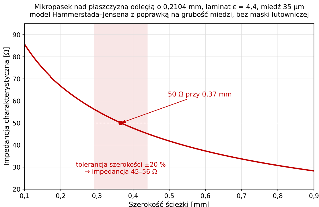
Rysunek 3. Impedancja charakterystyczna ścieżki mikropaskowej w funkcji jej szerokości, dla stosu czterowarstwowego z preimpregnatem 7628. Obliczenia według modelu Hammerstada–Jensena, dane materiałowe za tabelą stosów wytwórcy – jlcpcb.com/impedance
