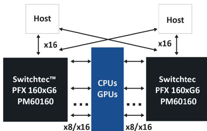
Rysunek 3. Przełączniki PCIe 6.0 typu fanout Switchtec PFX/PSX dzielą porty na łącza \times 8 i \times 16 . Przykład pokazuje, jak w typowym zastosowaniu w centrum danych przełączniki łączą wiele procesorów CPU i GPU przez łącza \times 16
