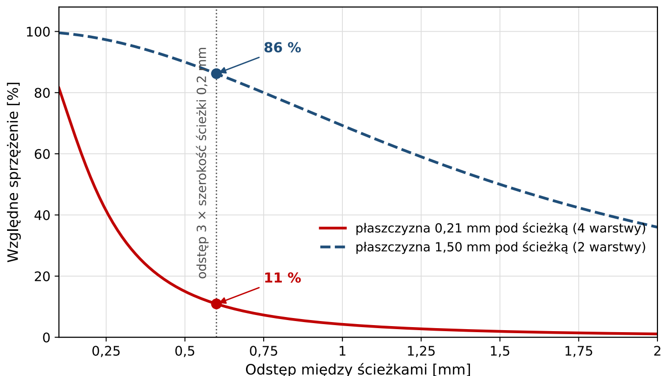
Rysunek 8. Sprężenie między sąsiednimi ścieżkami w zależności od odstępu, dla dwóch odległości od płaszczyzny odniesienia
