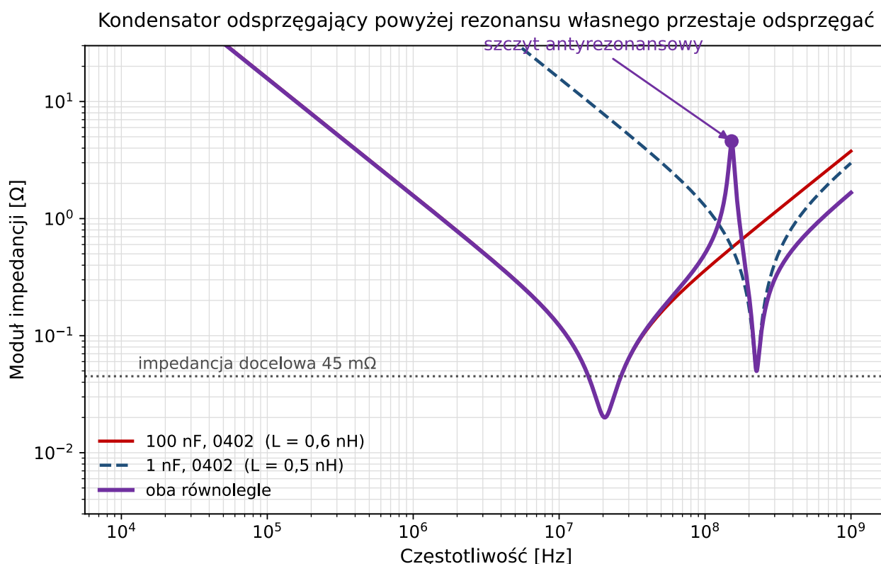
Rysunek 7. Impedancja kondensatora odsprężającego w funkcji częstotliwości oraz szczyt antyrezonansowy przy równoległym połączeniu dwóch wartości. Model szeregowy RLC z indukcyjnością montażu
