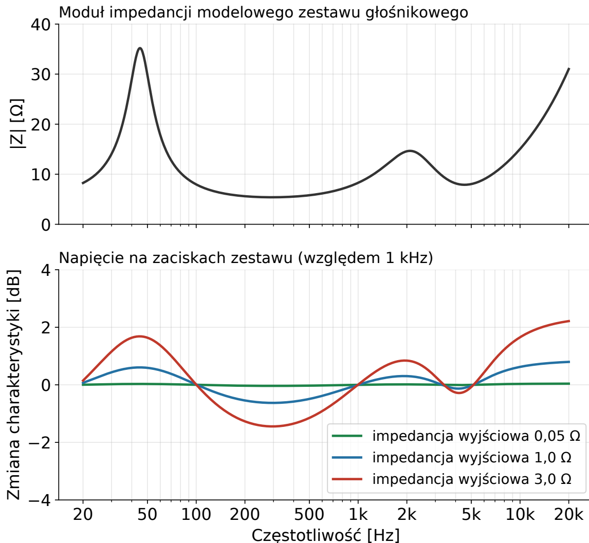
Rysunek 12. U góry: moduł impedancji modelowego zestawu dwudrożnego (rezonans 45 Hz, maksimum w okolicy podziału 2,2 kHz, minimum ok. 5,4 Ω). U dołu: zmiana napięcia na zaciskach zestawu względem wartości przy 1 kHz dla wzmacniacza o impedancji wyjściowej 0,05 Ω, 1 Ω i 3 Ω (obliczenia własne; model zestawu nie odpowiada żadnemu konkretnemu produktowi)
