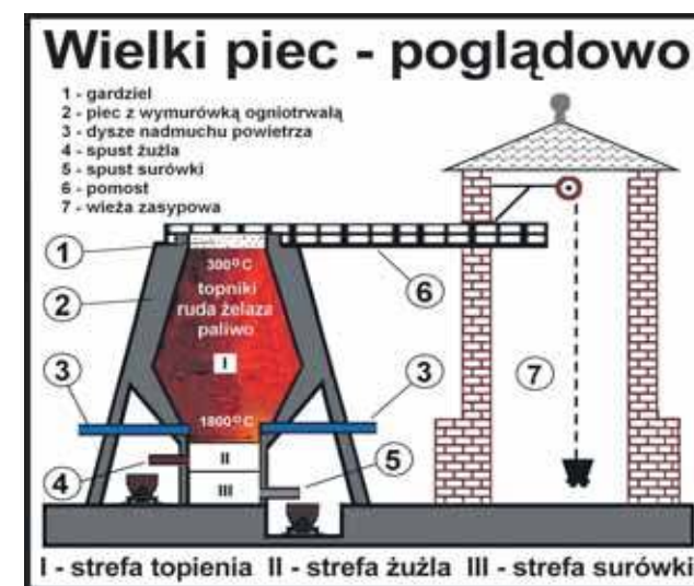
Schemat wielkiego pieca
