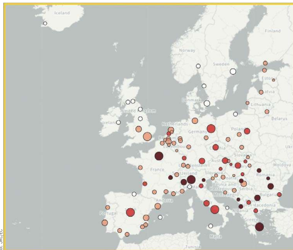
Intensywność miejskich wysp ciepła dla 100 miast UE
