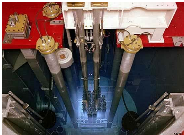
Fot. 3. Rdzeń reaktora jądrowego. Licencja Wikimedia Commons.
