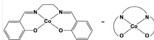
Rys. 1 Struktura salkominy
