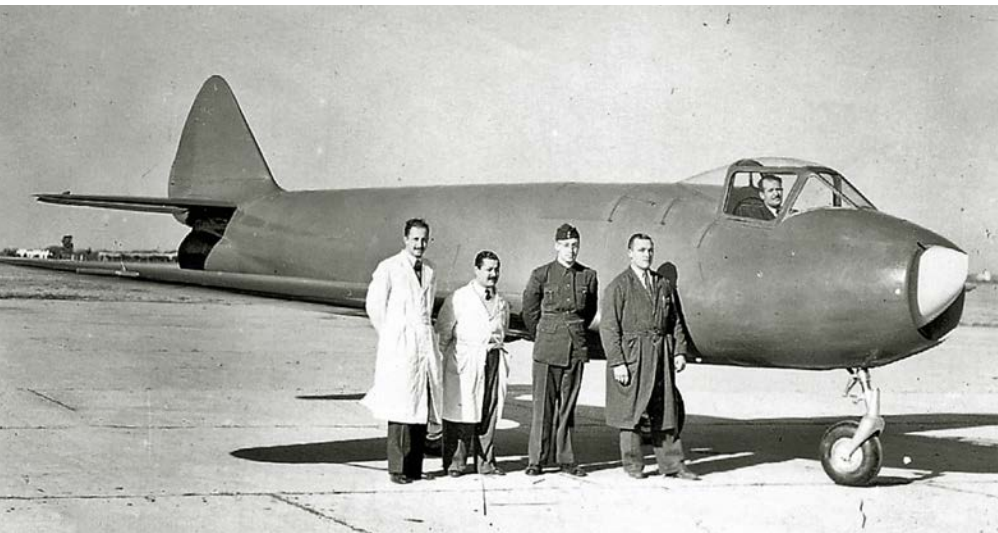
Inżynierowie opracowujący myśliwiec I.Ae.27 Pulqui (od lewej): Norberto Morchio, Eduardo Fernández, Humberto Ricciardi, Luis Mitchel i Enrique Cardeillac (w kokpicie). Samolot nie ma jeszcze namalowanego oznakowania ani zamontowanych pokryw przedniego podwozia.
