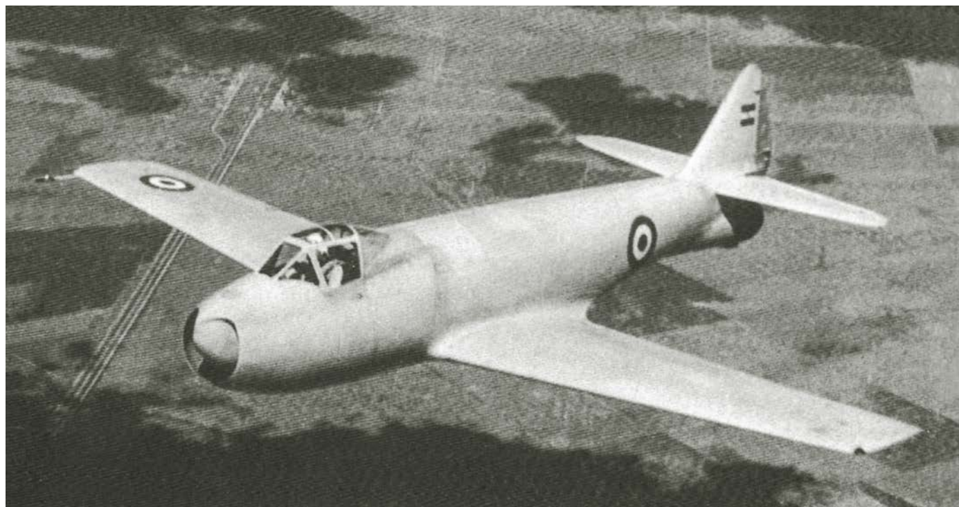
Zmodyfikowany prototyp I.Ae.27 Pulqui podczas jednego z nielicznych lotów próbnymi. Samolot ma już proste („ścięte”) końcówki skrzydeł. Prototyp Pulqui wykonał ostatni lot w marcu 1956 roku, a pod koniec 1960 został oficjalnie wycofany z eksploatacji.
