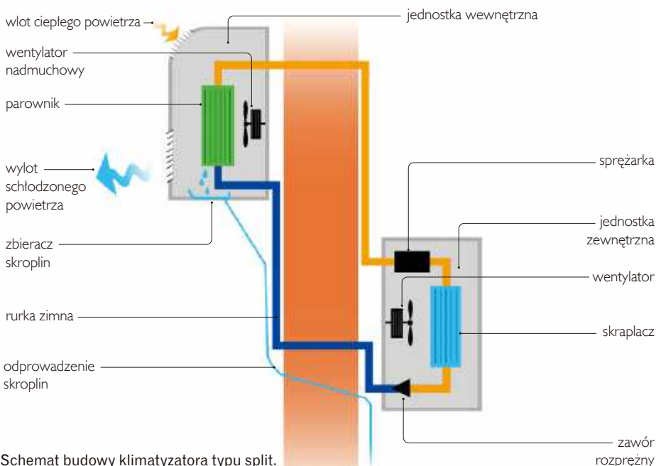
Schemat budowy klimatyzatora typu split.
