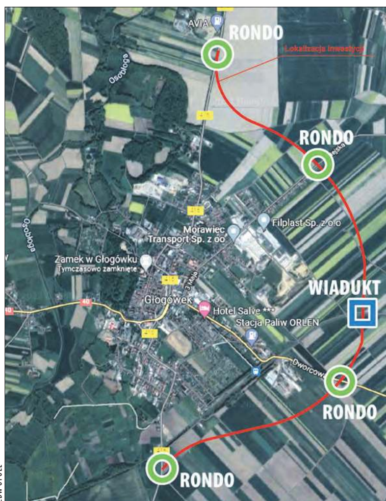
Koncepcja przebiegu obwodnicy miasta
