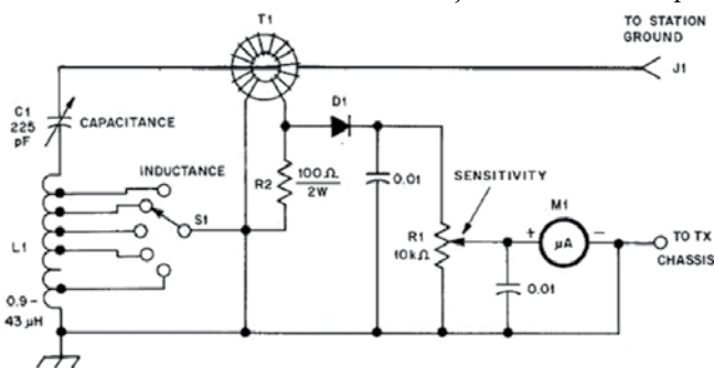
Rys. 1 Schemat układu MFJ-931
