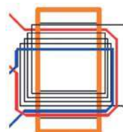
Rys. 8. Uzwojenie T3
