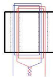
Rys. 6. Uzwojenie T1
