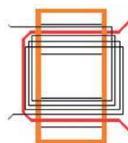
Rys. 7. Uzwojenie T2
