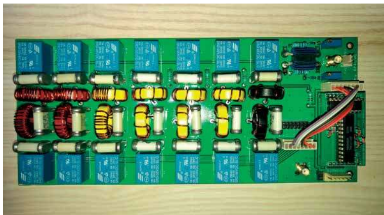
Płytki LPF wraz z modulem band dekodera już po zestrojeniu filtrów (wymiary płytki – 234×99 mm)
