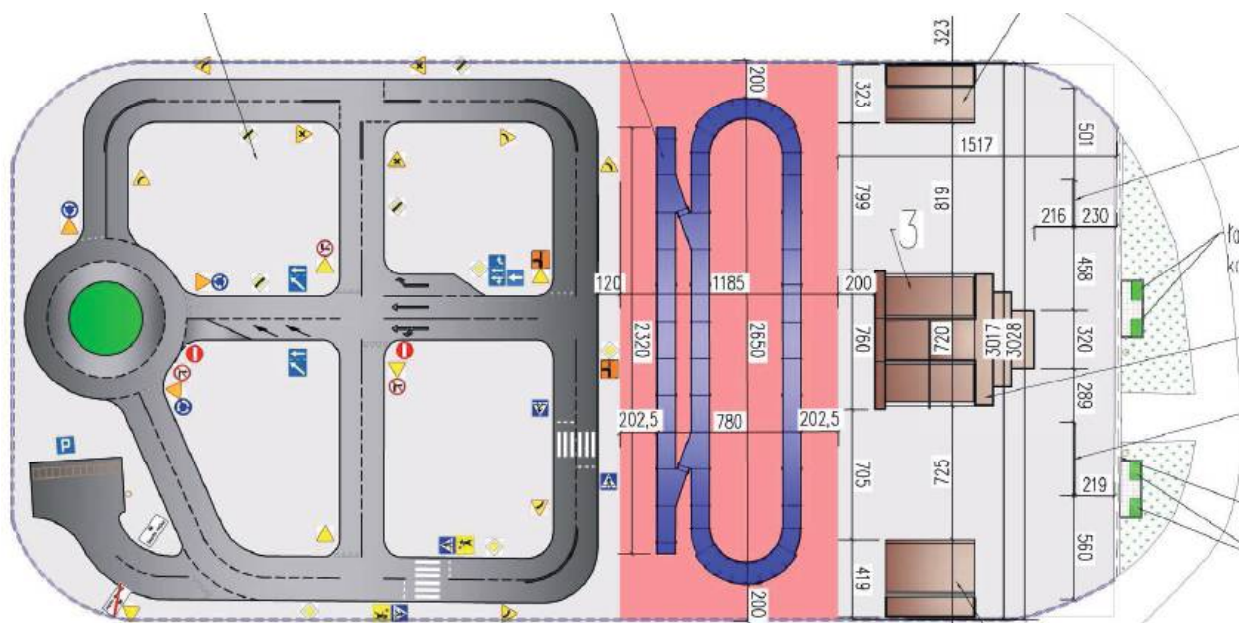
Projekt urządzenia skateparku (z prawej), toru rowerowego typu pumptrack (w środku na różowo) i miasteczka rowerowego do nauki jazdy (z lewej)
