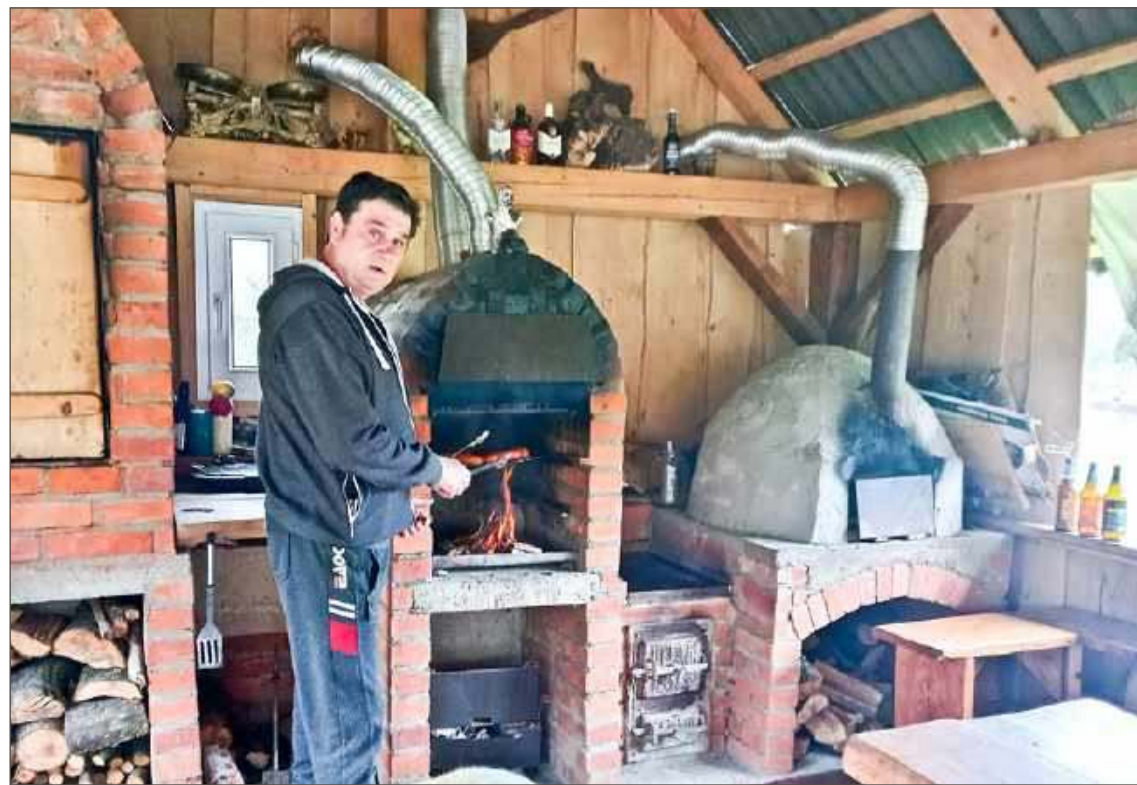
O takim grillu Krzysztof Świerk marzył, taki sobie sam zbudował.
