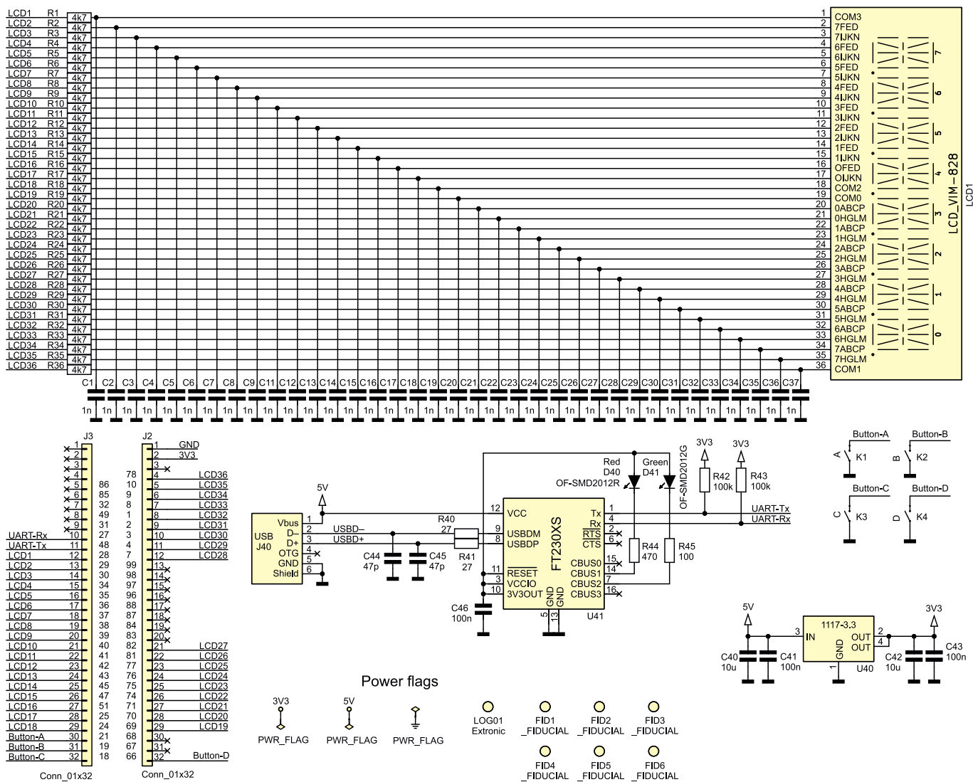
Rysunek 1. Schemat płytki
