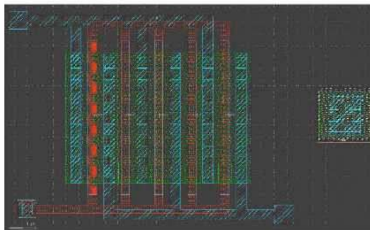
Rysunek 2. Przykład schematu opracowanego w Xschem oraz layoutu wykonanego z użyciem Klayout
