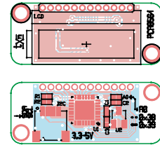
Rysunek 3. Rozmieszczenie elementów na płytce modułu (a – strona TOP, b – strona BOTTOM)
