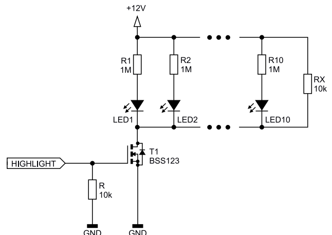
Rysunek 5. Modyfikacja uwzględniająca prąd zerowy drenu tranzystora sterującego
