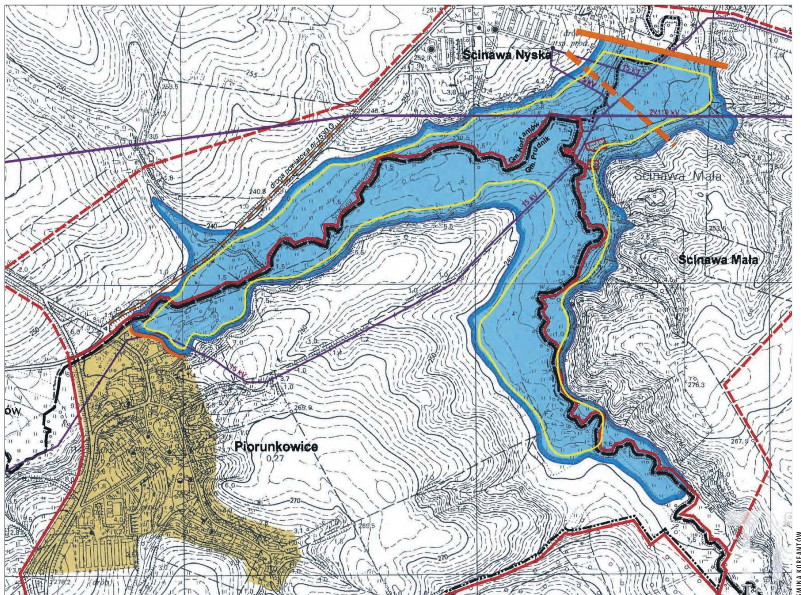
Koncepcja zbiornika Ścinawa – Piorunkowice
