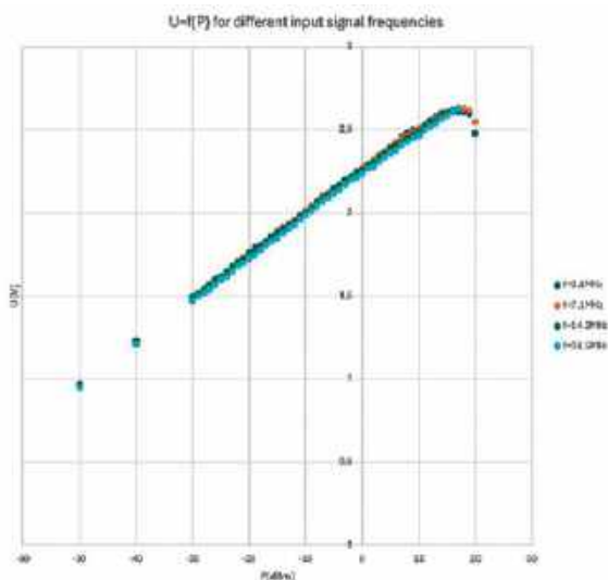
Rys. 1. Wykres zależności napięcia wyjściowego od poziomu mocy wejściowej dla układu AD8307
