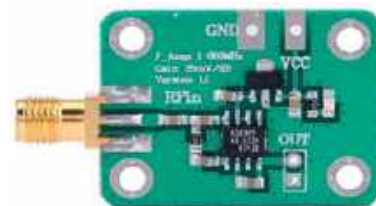
Rys. 2. Płytkę prototypową układu AD8307
