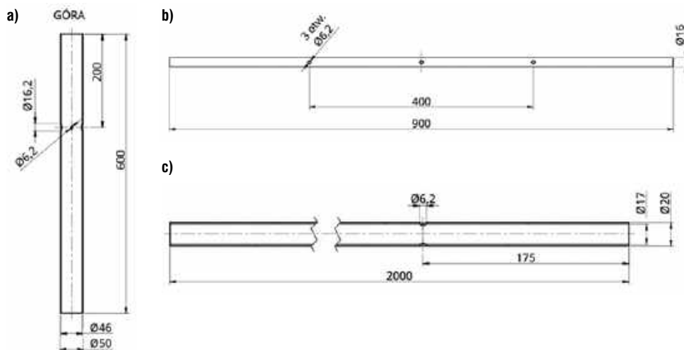
Rys. 4. Wymiary masytu (a), pręta mocującego bom (b) oraz rury tworzącej połowę bomu (c)
