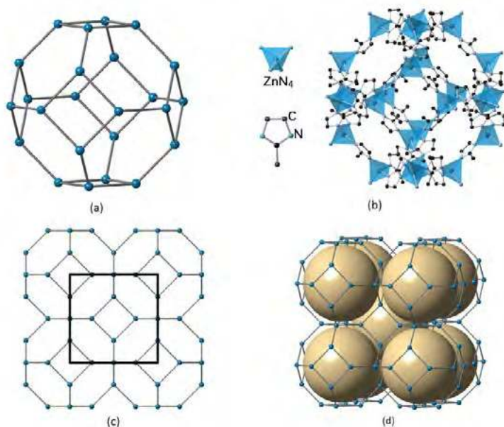
Rysunek 3.2 Topologia SOD i struktura ZIF-8: (a) Topologia klatki SOD; (b) Klatka SOD w ZIF-8 utworzona przez \text{Zn}^{2+} (w centrach tetraedrów) i imidazolan (atomy H pominięto dla przejrzystości); (c) Szkielet SOD z komórką elementarną pokazaną przez kwadratowe pole; (d) Niektóre pory w ZIF-8 są wyróżnione przez wirtualne kule.
