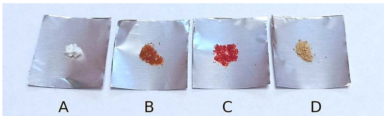
Fot. 1 – Chemiluminofores; A – lofina, B – lucygenina, C – heksahydrat chlorku tris(2,2'-bipirydylo) rutenu(II), D – luminol
