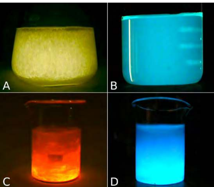
Fot. 2 – Chemiluminescencja; A – lofina (zielonożółta), B – lucygenina (zielononiebieska), C – chlorurek tris(2,2'-bipirydylo)rutenu(II) (pomarańczowoczerwona), D – luminol (niebieska)
