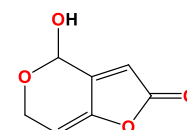
Rys. 4. Budowa cząsteczki patuliny.
