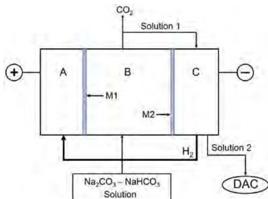
Rysunek 3.1 Schematyczny rysunek układu eksperymentalnego
