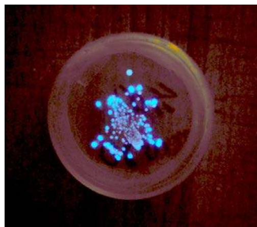
Fot. 3 – Bioluminescencja kolonii bakterii Aliivibrio fischeri na szalce Petriego z pożywką, czas ekspozycji: 5s, ISO:1000
