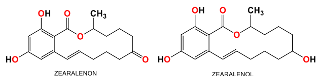
Rys. 7. Budowa cząsteczki zearalenonu (po lewej) i zearalenolu (po prawej).
