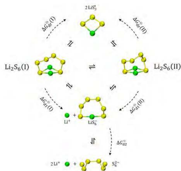
Równowagi chemiczne \text{Li}_2\text{S}_6 , \text{LiS}_6^- , \text{S}_6^{2-} i \text{LiS}_3^\bullet w DME
