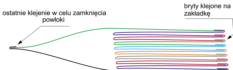
przekrój sklejonej powłoki balonu
