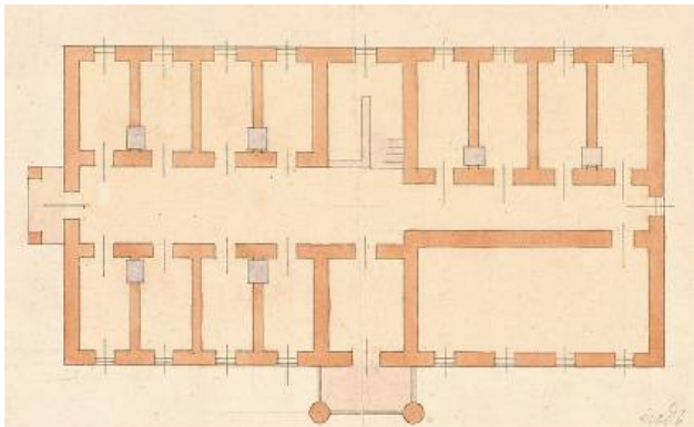
Plan „Rysunek budowli pozostałych po klasztorze Księży Bazylianów w mieście Chełmie, powiecie krasnostawskim, guberni lubelskiej” z 1865 r. (fragment), rzut piętra klasztoru Bazylianów, zbiory Archiwum Głównego Akt Dawnych w Warszawie
