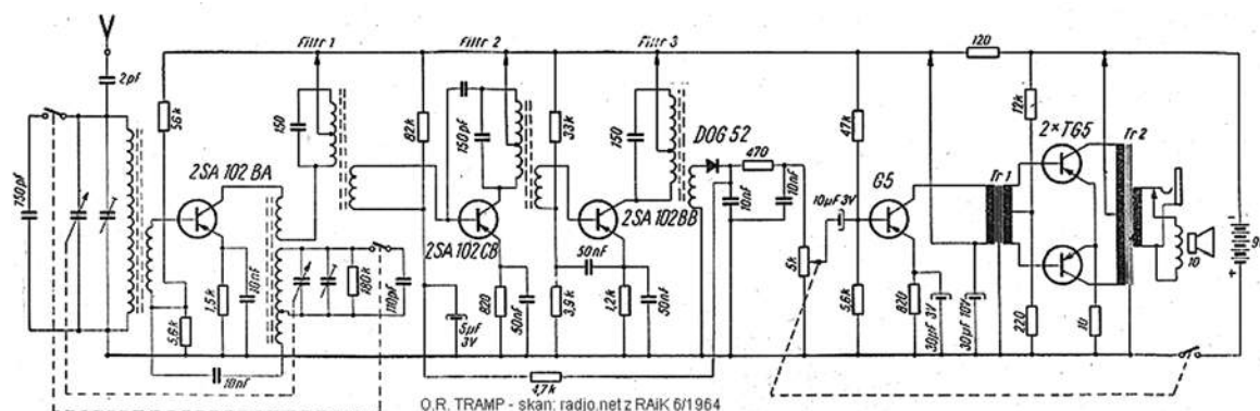
Rys. 1. Schemat ideowy odbiornika Tramp
