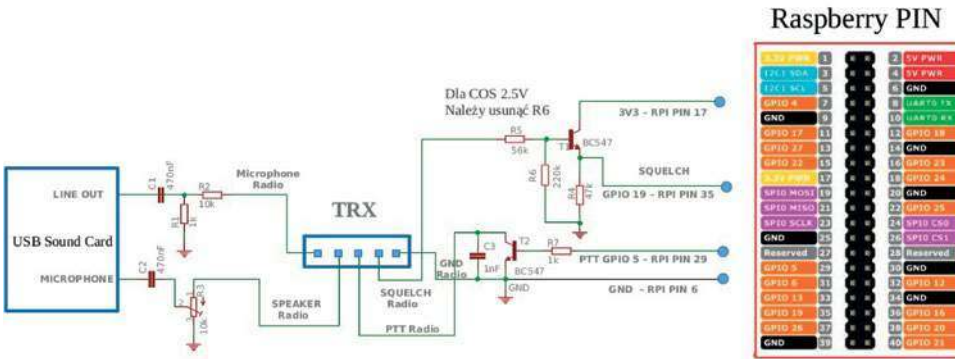
Rys. 6. Schemat podłączenia radia do Raspberry PI
