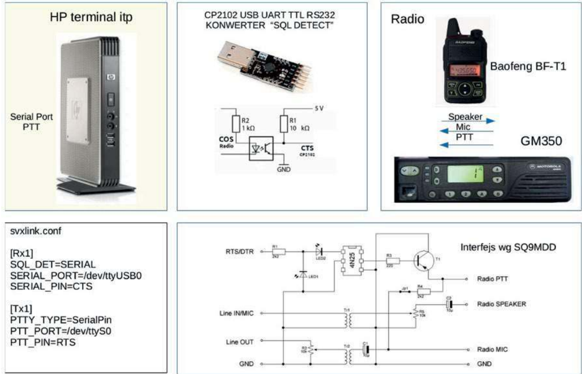
Rys. 4. Schemat podłączenia radia do terminalu PC HP
