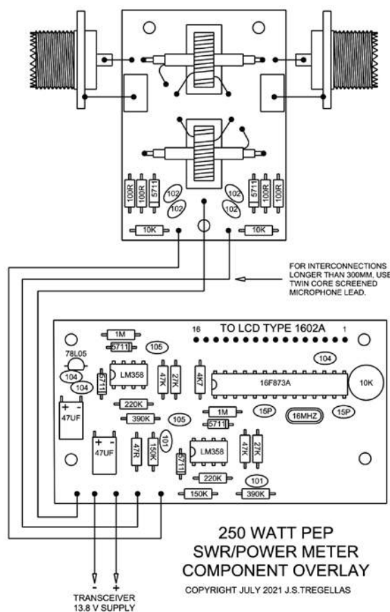
Rys.2. Rozmieszczenie elementów na płytkach drukowanych miernika
