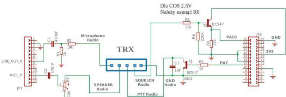
Rys. 5. Schemat podłączenia radia do Orange PI ZERO (v1.x)
