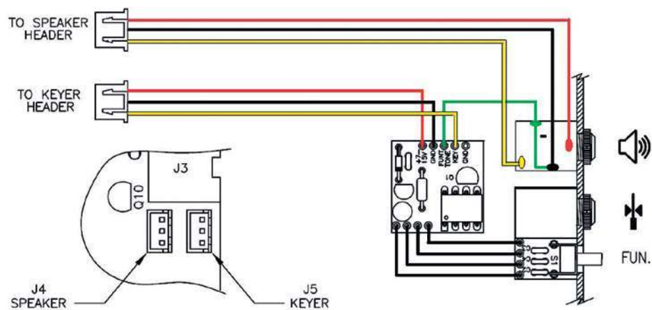
Rys. 4. Sposób podłączenia oddzielnych gniazd DSB i CW
