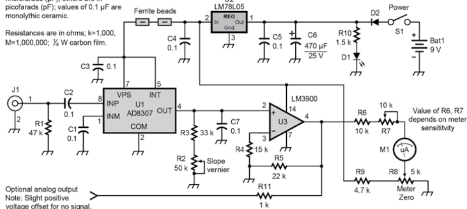
Rys. 3. Schemat miernika natężenia pola elektromagnetycznego
