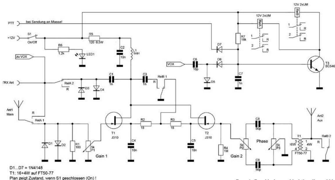
Rys. 1. Przykładowy układ tłumika zakłóceń
