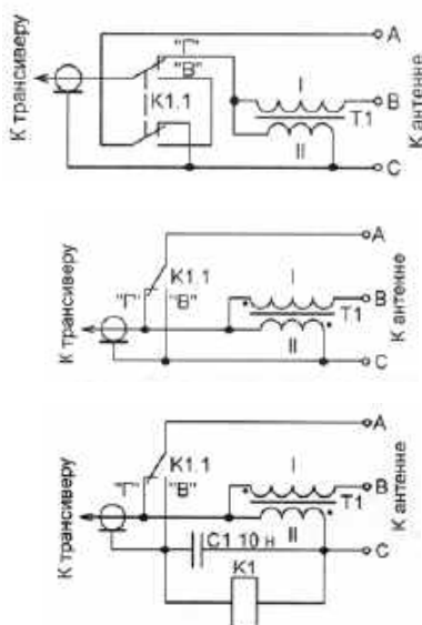
Rys. 3. Schematy różnych sposobów przełączania polaryzacji anteny
