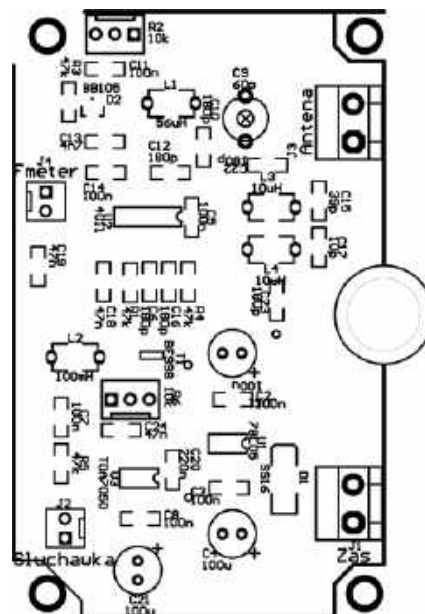
Rys. 3. Rozmieszczenie elementów na płytce
