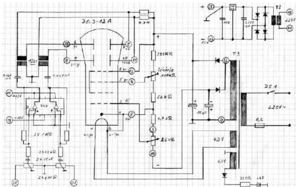
Rys. 5. Przykładowy schemat układu dostrojenia do sygnału RTTY z lampą oscyloskopową
