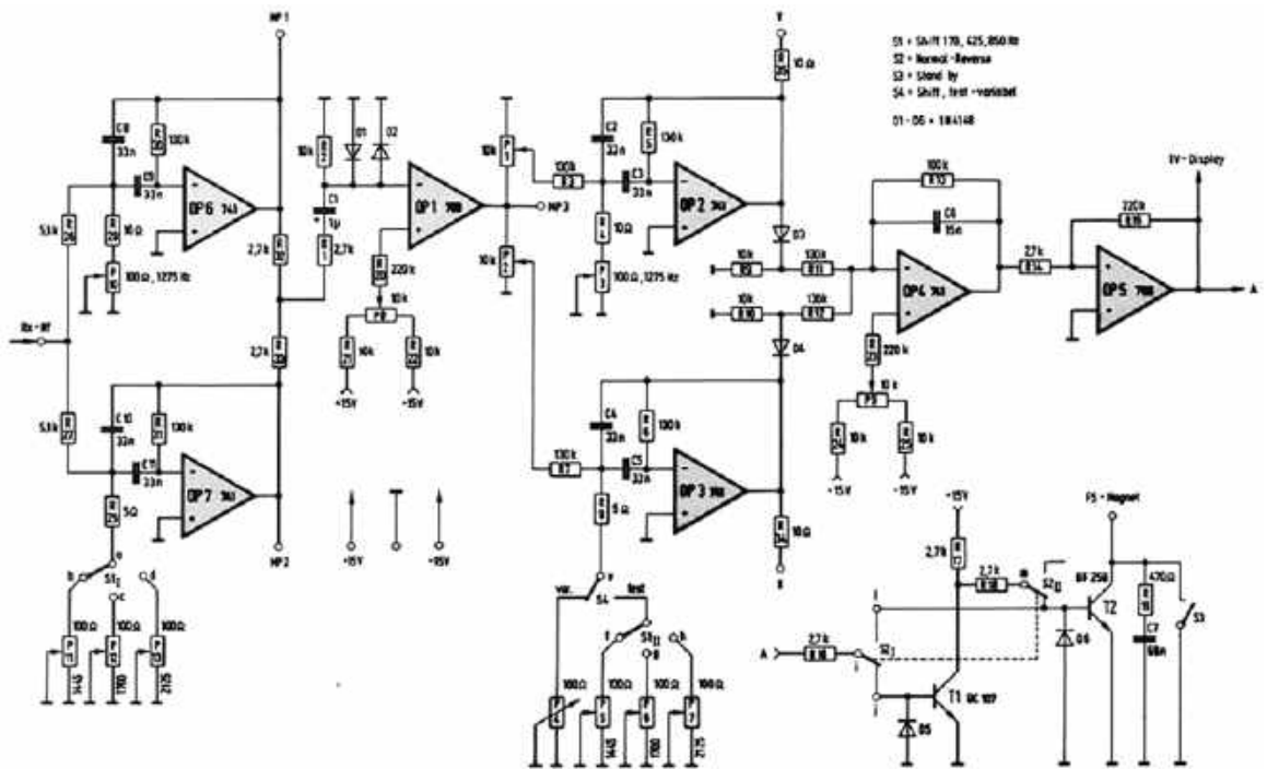
Rys. 4. Schemat konwertera do RTTY według DJ6HP
