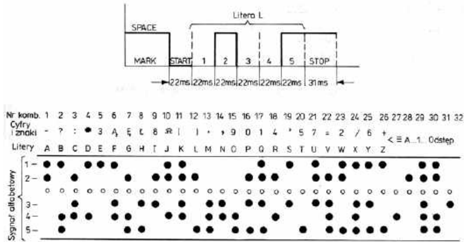
Rys. 1. Impulsy telegraficzne RTTY
