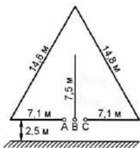
Rys. 2. Szkic anteny Delta 40 m wg RN3KV
