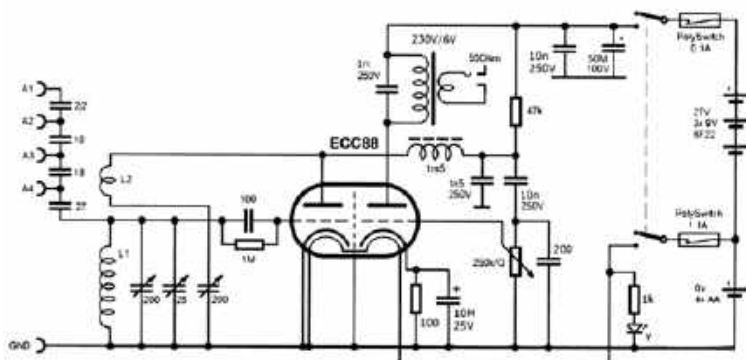
Rys. 1. Schemat lampowego odbiornika reakcyjnego
