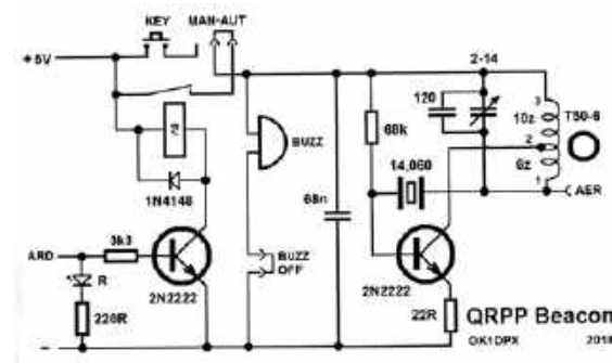
Rys. 2. Schemat nadajnika QRPP (radiolatarnia na pasmo 20 m)
