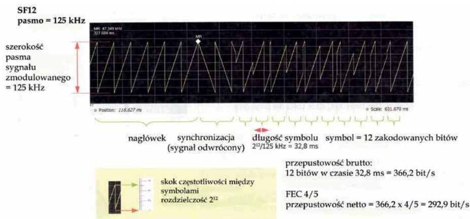
Rys. 2. Sygnał systemu LoRa zmierzony analizatorem widma (źródło: „Elektron” 5-6/2017). Pod białym wskaźnikiem rozpoczyna się nagłówek komunikatu
