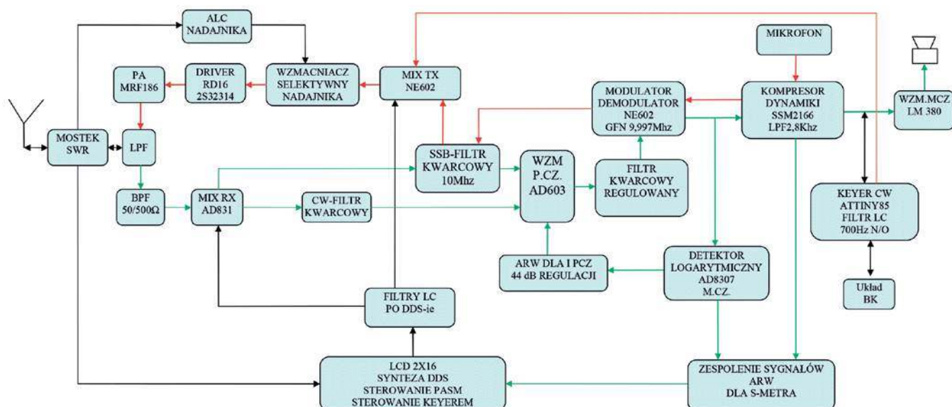
Rys. 1. Schemat blokowy transceivera Hydra
