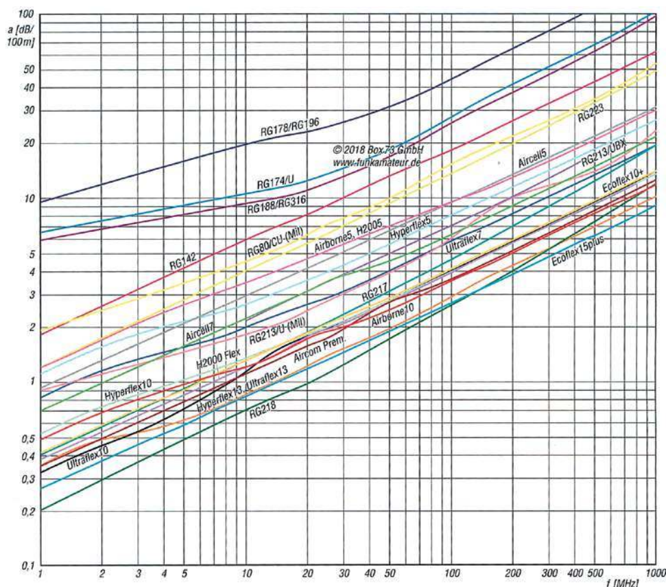
Rys. 2. Charakterystyka amplitudowo-częstotliwościowa tłumienia różnych kabli na odcinku 100 m w zakresie od 1 do 1000 MHz (źródło: „Funk Amateu” 5/2018)
