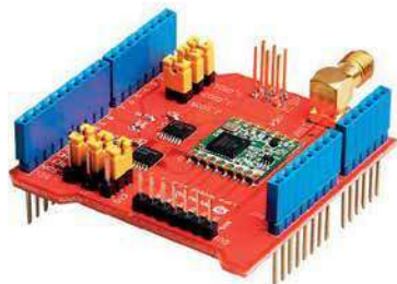
Moduł Dragino dla Arduino UNO, Mega (2560), Due i Leonardo
