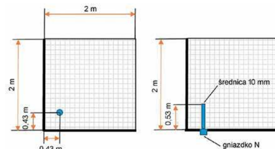
Rys. 9. Wymiary anteny IW5BHY
