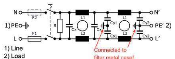
Rys. 4. Schemat ideowy filtra sieciowego zaczerpnięty z Internetu
