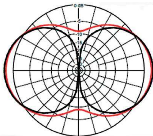
Rys. 2. Charakterystyka promieniowania w płaszczyźnie pionowej. Linia czarną przedstawiono wyniki symulacji dla szczeliny prostej, a czerwoną – dla załamanej
