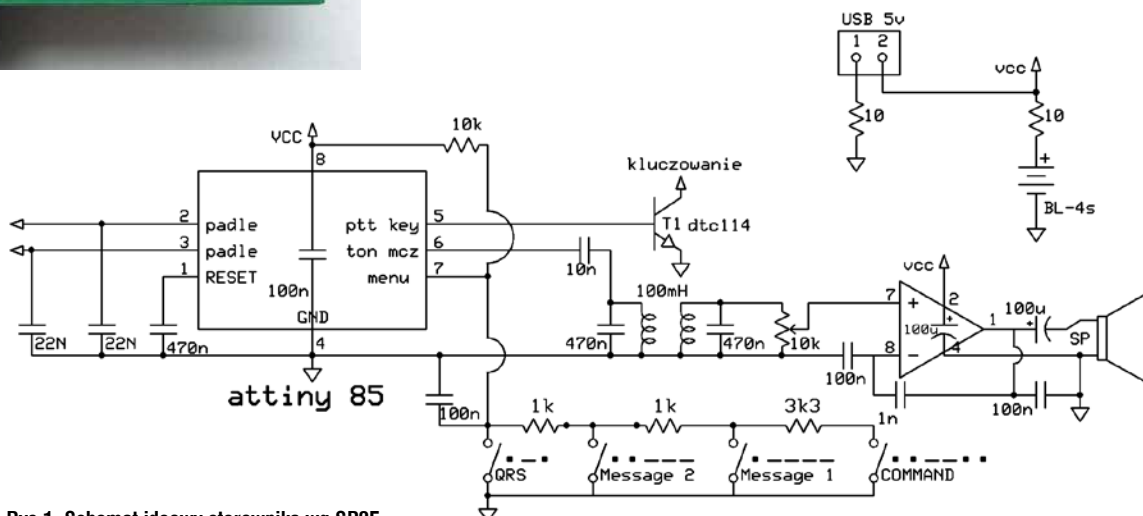
Rys 1. Schemat ideowy sterownika wg SP2F
