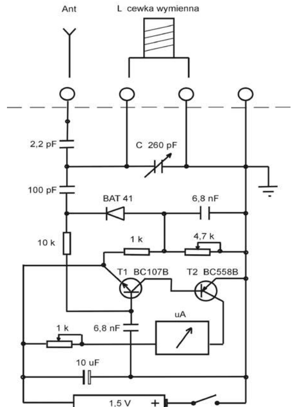
Rys. 3. Schemat ideowy falomierza wg SP20FS
