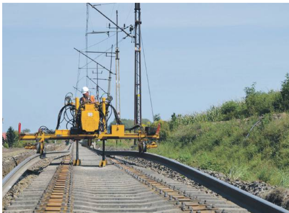
Specjalistyczna maszyna do przesuwania szyn
