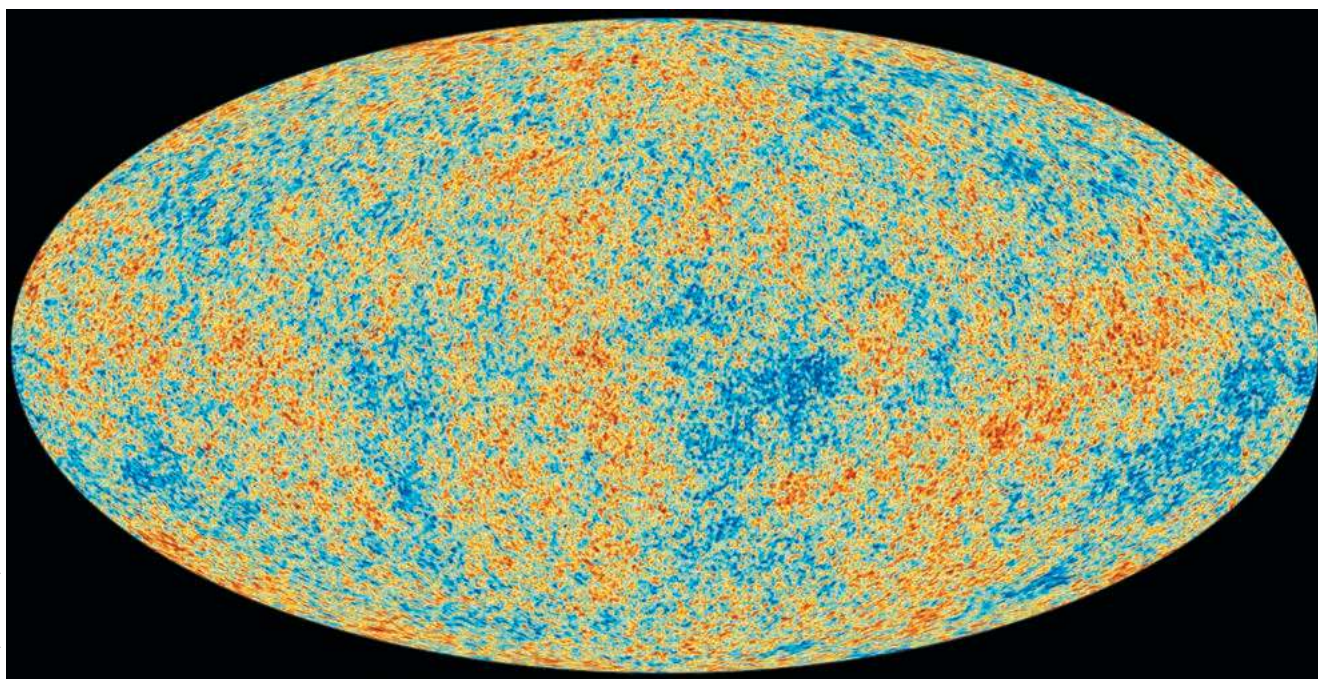
Mapa temperatury mikrofalowego promieniowania tła wykonana przez satelitę Planck. To „luna po Wielkim Wybuchu”. Różnice w kolorach (temperaturze) odpowiadają niewielkim wahaniom gęstości materii we wczesnym wszechświecie. Dały one, za sprawą siły grawitacji, początek gromadom galaktyk.
