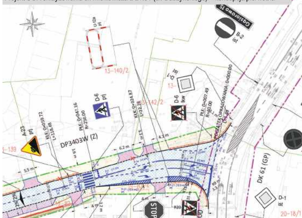
Projekt SOR skrzyżowania ul. Mickiewiczza z DK61 (ul. Daszyńskiego) – koncepcja pierwotna
