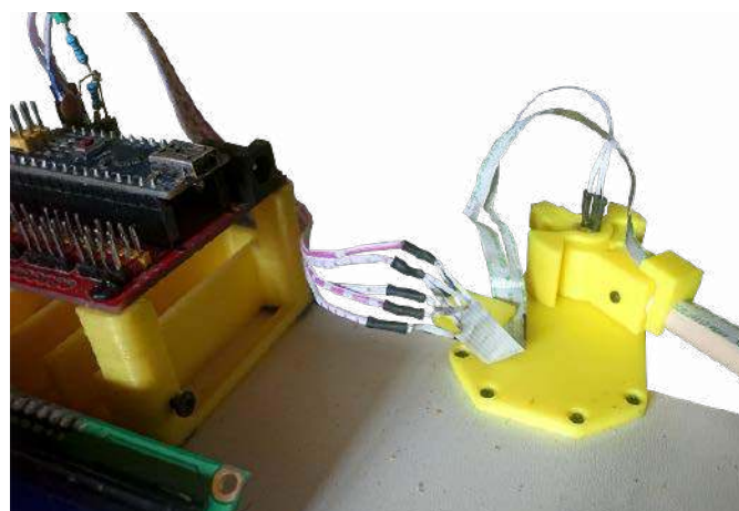
Fotografia 1. Wiązka łącząca ramię z płytą i modułem Arduino
