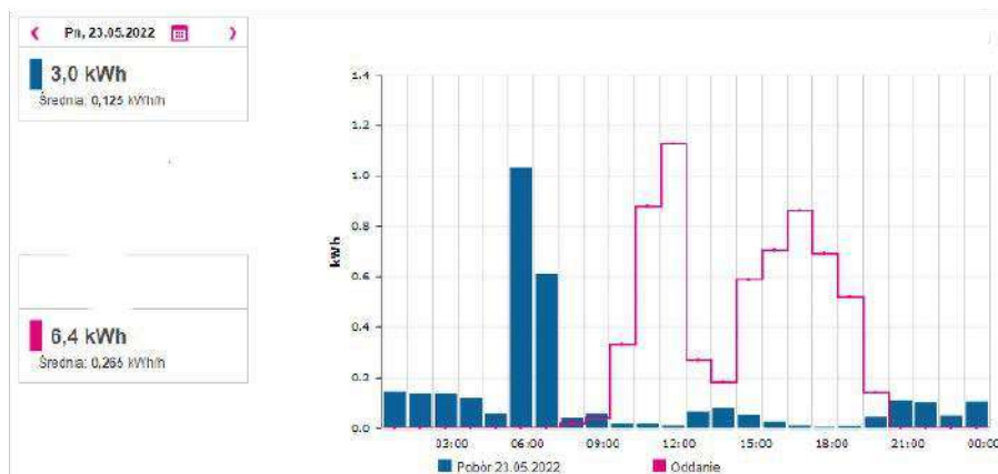
Rysunek 1. Wykres pokazujący przerwy w oddawaniu energii do sieci, które występują w momencie największego nasłonecznienia
