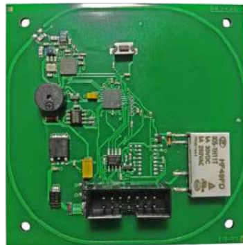
Fotografia 9. Moduł CTU-R5RM marki Netronix ( https://bit.ly/3Ak0s3n )
