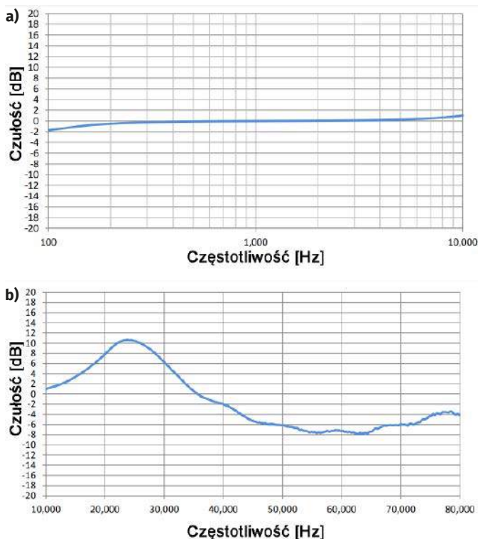
Rysunek 4. Charakterystyka częstotliwościowa mikrofonu SPH0641LU4H-1: a) zakres akustyczny, b) zakres ultradźwiękowy
