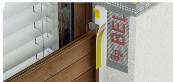
BP13 R LISTWA DYLACYJNA DO PRÓWADNIC ROLET W SYSTEMACH ROLET OKIENNYCH ZEWNĘTRZNYCH
