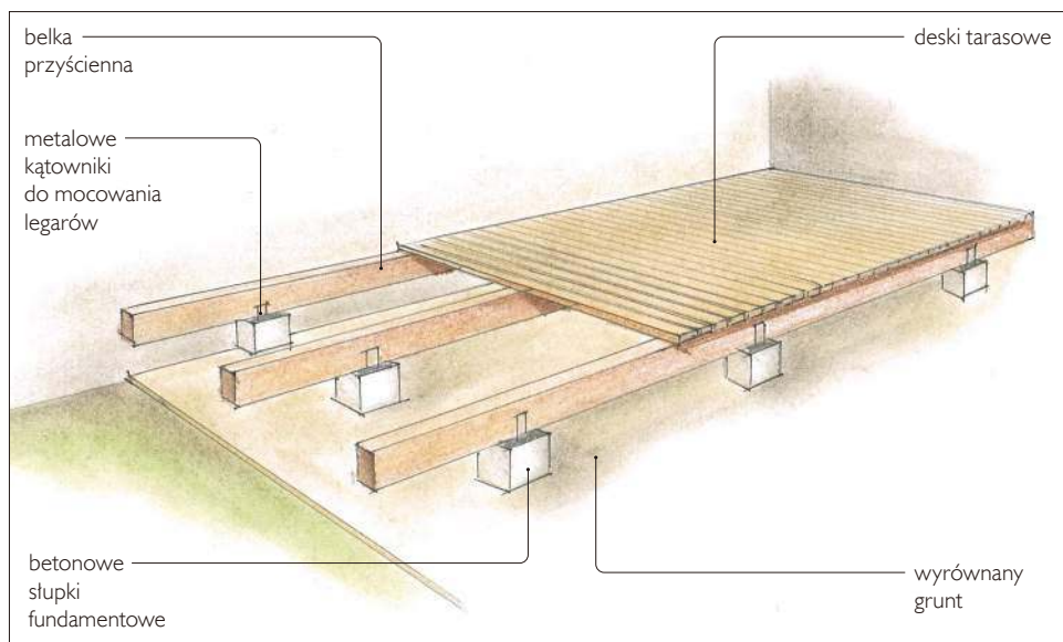
📍 Sposób wykonania tarasu drewnianego na betonowych podporach.
