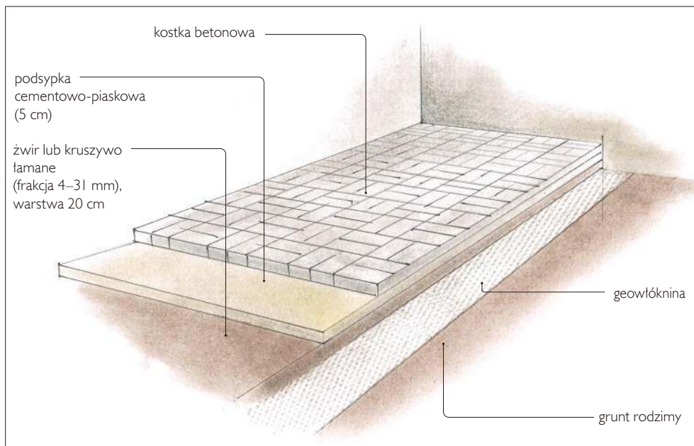
❶ Sposób wykonania tarasu na gruncie wykończonego kostką betonową.
