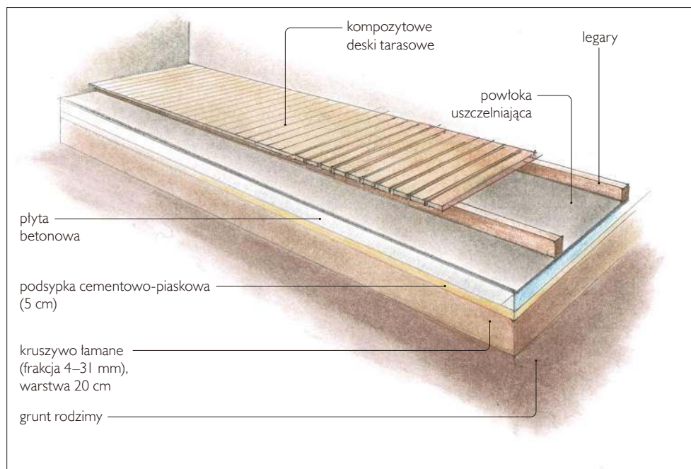
📌 Sposób wykonania tarasu z desek kompozytowych.
