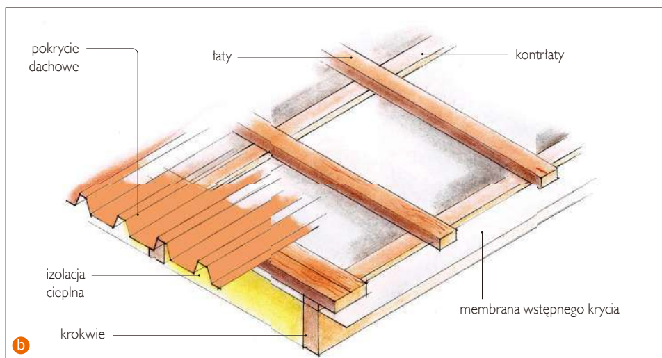
🔧 Podkład dachowy może mieć formę deskowania (a) lub ołaceń (b).
