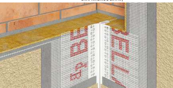
BP16 V LISTWA PVC DYLACYJNA TYPU „V” - KĄTOWA Z SIATKĄ
