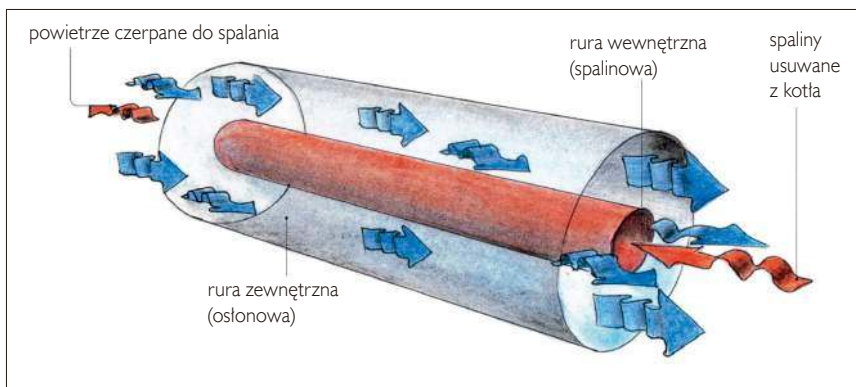
🔗 Zasada działania koncentrycznego przewodu powietrzno-spalinowego.
