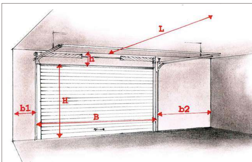
🔑 Najważniejsze pomiary, które trzeba wykonać przed zakupem bramy: szerokość i wysokość otworu wjazdowego (B i H); szerokość ścianek bocznych – odległość między ścianą boczną, a otworem wjazdowym (b1 i b2); wysokość nadproża (h); głębokość garażu – wolna przestrzeń pod sufitem (L).
