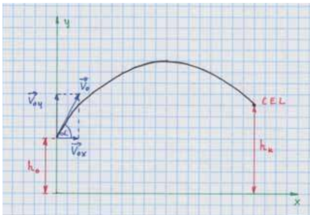
Rys. 1. Tor ruchu strzały wystrzelonej z łuku z prędkością początkową v_0 .
