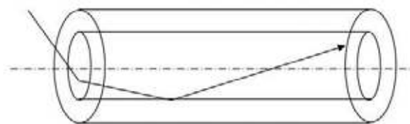
Rys. 4. Przebieg promienia ukośnego.
