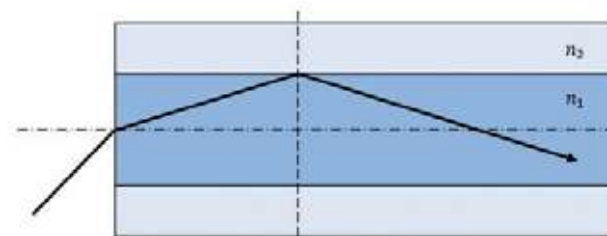
Rys. 3. Przebieg promieni południkowych (w rzucie planarnym).
