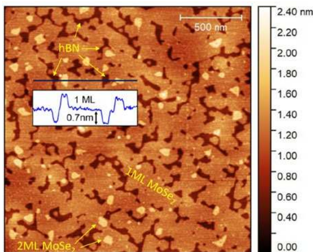
Rys. 6 Obraz z mikroskopii sił atomowych pozwala uwidocznić strukturę powierzchni dichalkogenu \text{MoSe}_2 . Ciemnopomarańczowe obszary to podłoże h-BN, jasnopomarańczowe – warstwy o grubości pojedynczej cząsteczki \text{MoSe}_2 (1 ML), natomiast żółte – dwuwarstwy \text{MoSe}_2 (2 ML). Zaprezentowano również zmianę topografii powierzchni wzdłuż grubej granatowej linii. Obrazek pochodzi z publikacji [4].
