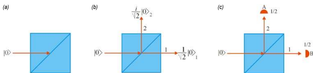
Rysunek 1. (a) Foton padający na płytkę światłodzielącą PSD. (b) Za PSD foton znajduje się w stanie będącym superpozycją stanu po przejściu na wprost i po odbiciu. (c) Pomiar niszczy superpozycję. Stan fotonu kolapsuje z jednakowym prawdopodobieństwem 1/2 do jednego z dwóch stanów. Foton jest rejestrowany tylko przez jeden detektor.
