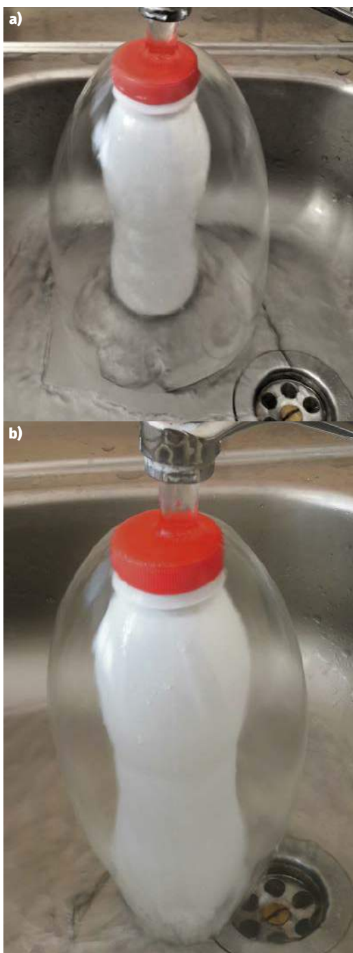
9. Zakrzywienie dolnej powierzchni „parasola wodnego” w kierunku osiowym w zależności od prędkości wypływu: a) kształt zbliżony do powierzchni paraboloidy, b) kształt bardziej przypominający fragment powierzchni elipsoidy. Efekt uzyskano w wyniku rozprętu wody po odrzucie hydraulicznym na zakrętce plastikowej butelki od kefiru
