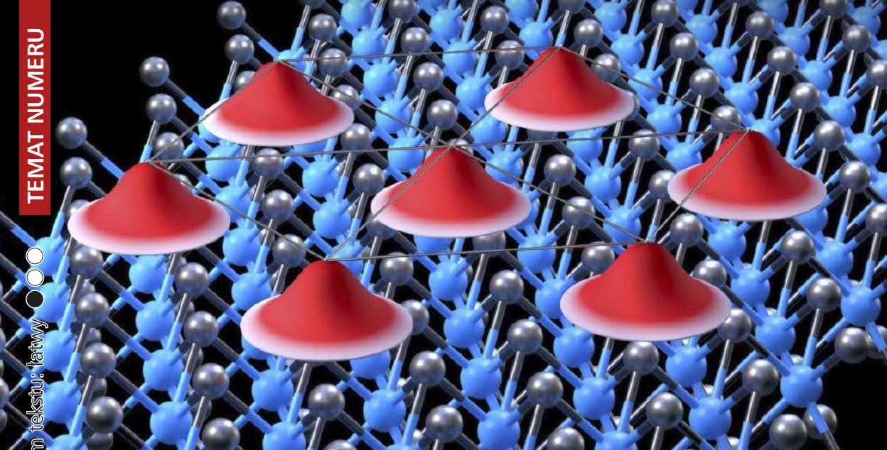
1. Kryształ Wignera wykonany z elektronów
