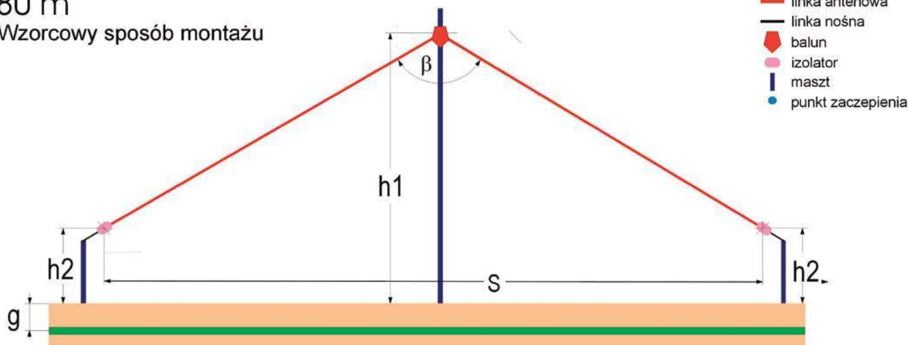
Rys. 1. Warunki wykonywania pomiarów anteny FR-1803
