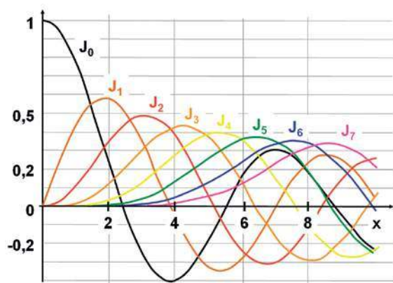
Rys. 11. Przebieg funkcji Bessela niższych rzędów. Funkcja J_0 przedstawia zależność amplitudy fali nośnej od indeksu modułacji, J_1 – zależność amplitudy pierwszej pary prążków, J_2 – drugiej itd.
