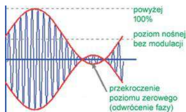
Rys. 4. Przeładowanie amplitudy. W miejscach przeładowania powstaje nośna o odwróconej fazie
