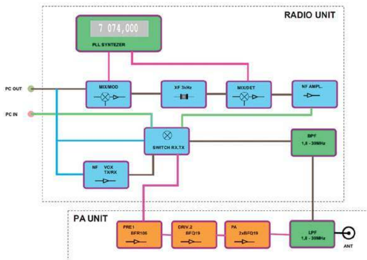
Rys. 1. Schemat blokowy Niki2
