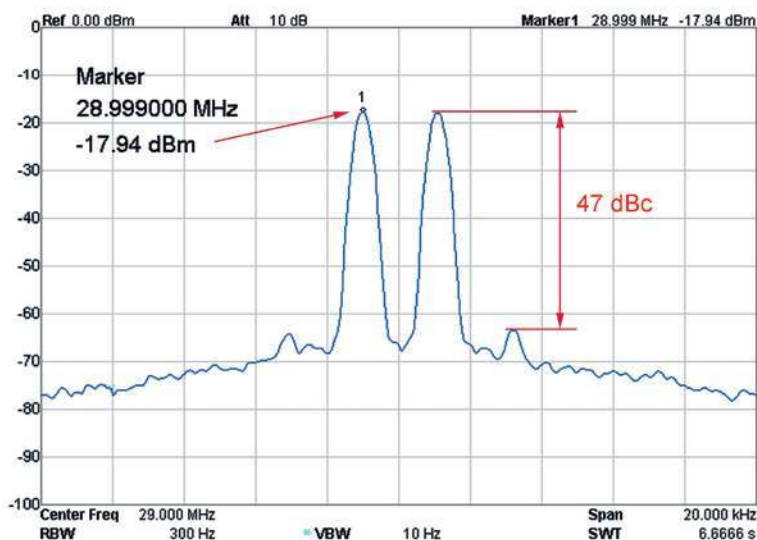
Rys. 3. Widmo sygnału p.cz. 28 MHz
