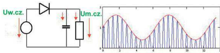
Rys. 6. Demodulator obwiedni. Dioda obcina dolne połówki zmodulowanej nośnej, resztki prądów w.c.z. są zwierane przez kondensator, a na oporniku odkłada się napięcie m.c.z.
