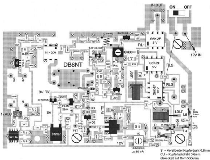
Rys. 4. Rozmieszczenie elementów na płytce transwertera
