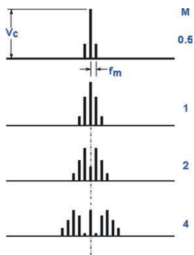
Rys. 10. Widma sygnału zmodulowanego częstotliwościowo pojedynczym tonem dla różnych indeksów modulacji. Dla indeksu mniejszego od jedności widmo zawiera dwa prążki, prążków przybywa w miarę zwiększania indeksu modulacji. Na rysunku przedstawiono wartości bezwzględne napięć bez uwzględnienia różnicy faz. Prążki wstęgi dolnej są zawsze odwrócone w fazie o 180 stopni w stosunku do górnej
