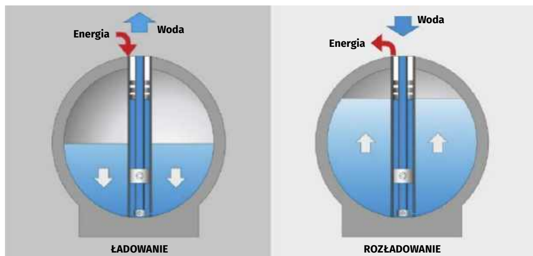
10. Zasada podwodnego magazynowania energii
