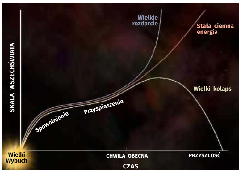
3. Scenariusze przyszłości Wszechświata
