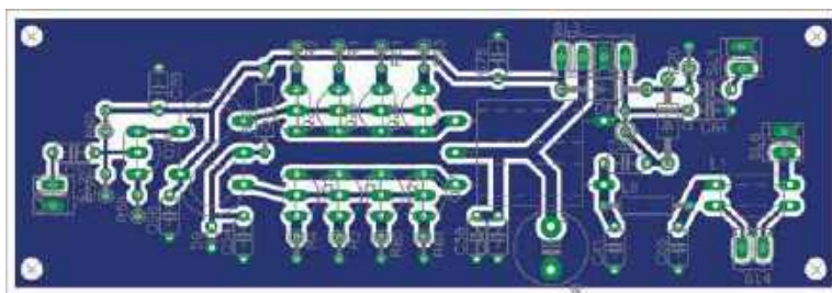
Rys. 6. Płytkę modułu PA i rozmieszczenie elementów na PCB
