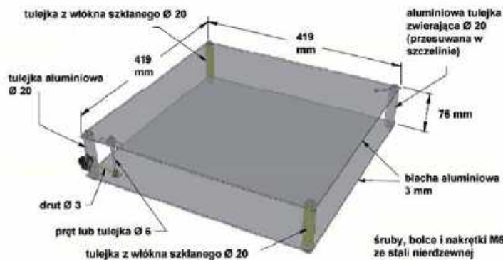
Rys. 1. Konstrukcja anteny
