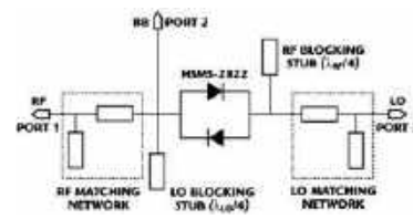
Rys. 4. Zasada działania miksera harmonicznych
