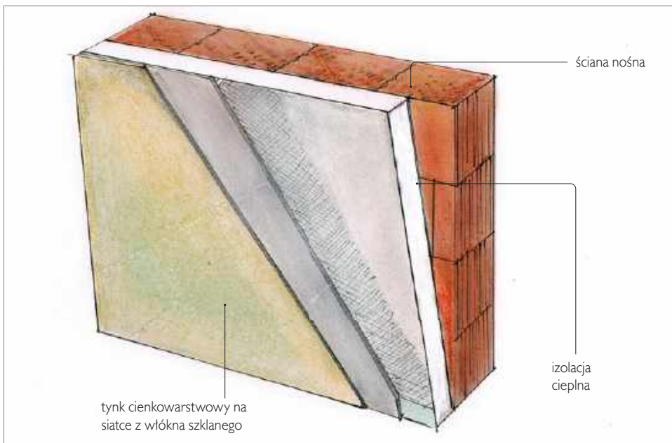
❶ Schemat ocieplenia ściany metodą lekką mokrą.
