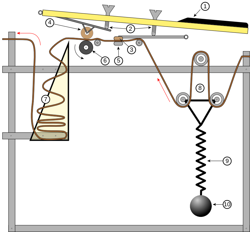
Rysunek 3. Schemat mechanizmu Mellotronu. Naciśnięcie klawisza (1) powoduje, że dwie śruby (2) łączą płytkę dociskową (3) z głowicą taśmy (5) oraz koło dociskowe (4) z obracającym się w sposób ciągły wałkiem napędowym (6). Taśma jest naciągana ze stałą prędkością, równoważona sprężyną naciągową (8...10) i tymczasowo przechowywana w pojemniku (7) do momentu zwolnienia klawisza
