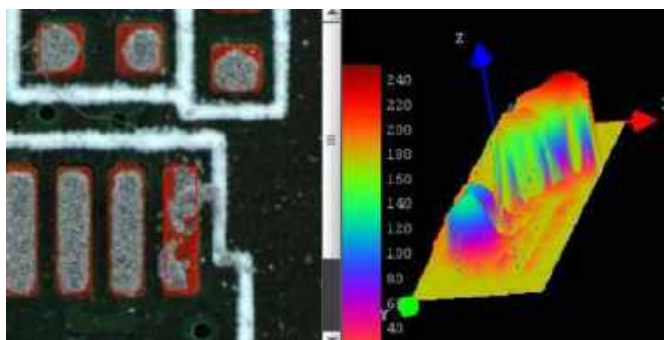
Fotografia 3. Przykładowy obraz z kamery maszyny SPI oraz render trójwymiarowy błędnie nałożonej pasty lutowniczej ( https://t.ly/qIXGp )
