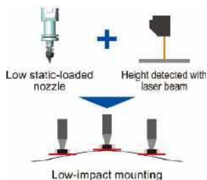
Rysunek 1. Zastosowanie laserowego skanera głębi do wspomagania montażu najmniejszych elementów SMD w automatach marki Yamaha ( https://t.ly/DmMWC )
