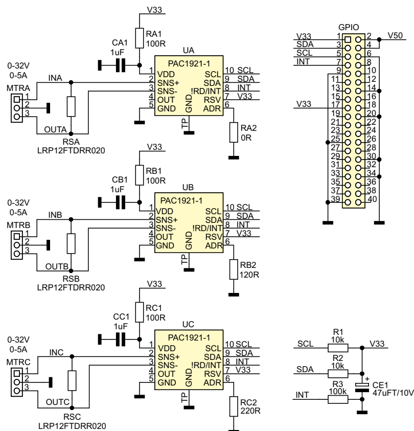
Rysunek 2. Schemat ideowy układu
