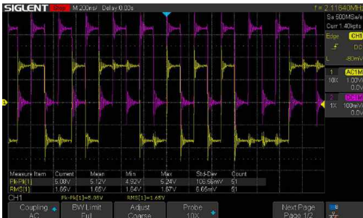
Rysunek 1. Zrzut ekranu z oscyloskopu demonstrujący sygnały wygenerowane przez Tang Primer 25k
