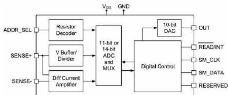
Rysunek 1. Budowa układu PAC1921 (za notą Microchip)
