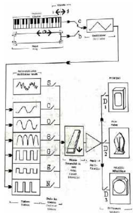
Rysunek 2. Schemat blokowy fal Martenota
