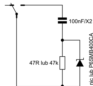
Rysunek 2. Stosowany przeze mnie obwód gaszący RCD
