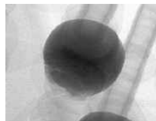
Fotografia 19. Obraz rentgenowski pokazujący uszkodzenie kulki spoina pod układem BGA. Widok zarejestrowany przy użyciu systemu MXI QUADRA 7 Pro ( https://t.ly/VH_x )
