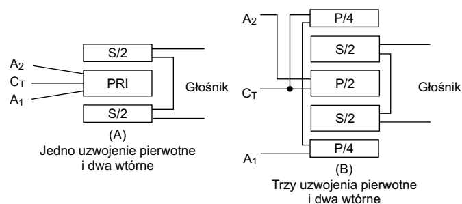
Rysunek 1. Układ uzwojeń na karkasie z dwóch wersji sekcjonowania [3]
