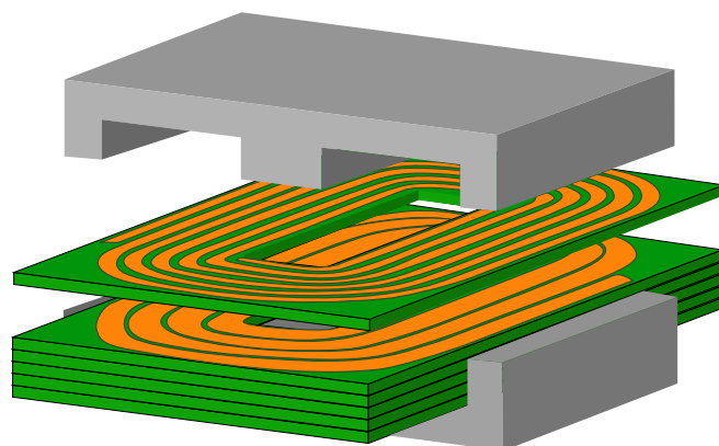
Rysunek 5. Budowa transformatora planarnego z użyciem PCB [10]
