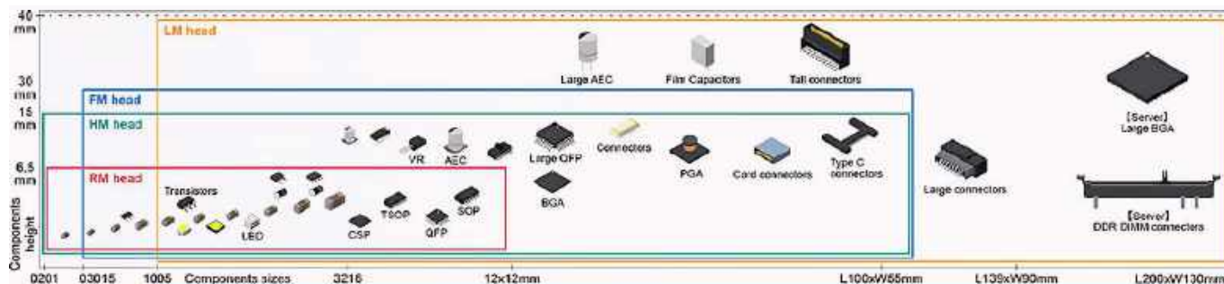
Rysunek 2. Zakres rozmiarów komponentów montowanych przez poszczególne głowice przeznaczone do automatów YRM20DL marki Yamaha ( https://t.ly/DmMWC )
