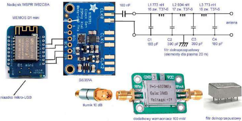
Rys. 2. Nadajnik WB2CBA. Na proponowane przez OE1KDA dodatki składają się wzmacniacz o mocy wyjściowej 100 mW (konieczne jest obniżenie mocy sterującej z syntezy do ok. 1 mW za pomocą tłumika) i fabryczny filtr dolnoprzepustowy
