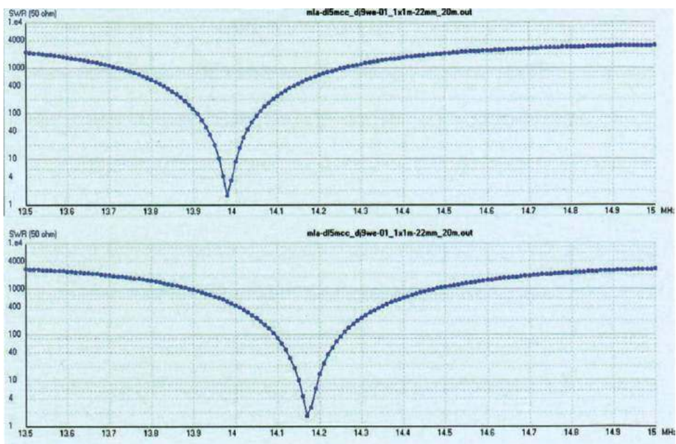
Rys. 6. Przykładowy przebieg WFS dla pętli maksymalnie sprzężonych (równoległych) u góry i rozchylonych – u dołu
