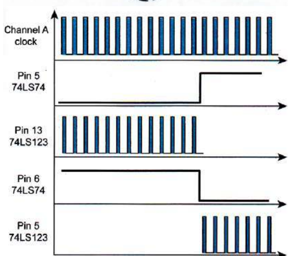
Rys. 5. Sposób formowania impulsów w enkoderze
