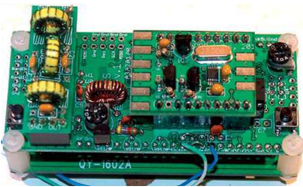
Fot. 3. Ultimate 3S od tyłu, na środku widoczna płytka syntezy Si5351A a po lewej stronie płytka filtra dolnoprzepustowego. Dół stosu stanowi płytka z niewidocznym od tej strony wyświetlaczem
