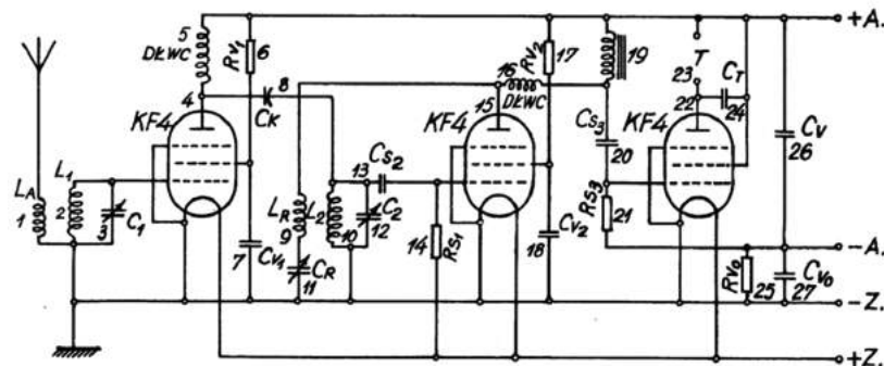
Rys. 5. Schemat ideowy odbiornika OBAr
