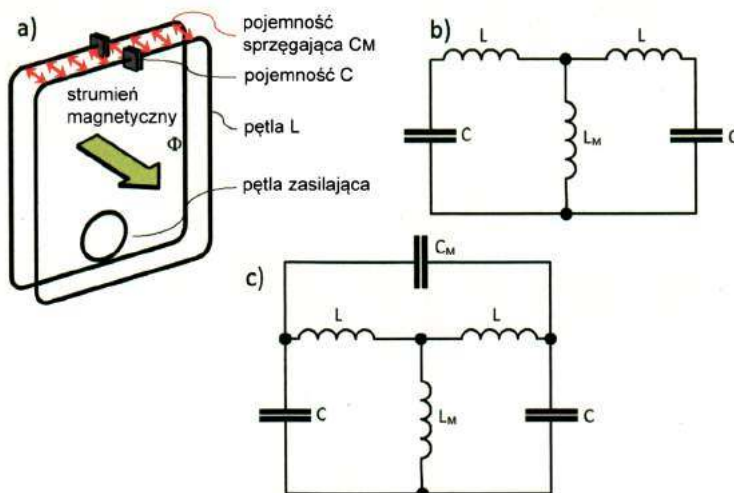
Rys. 2. Schematy zastępcze
