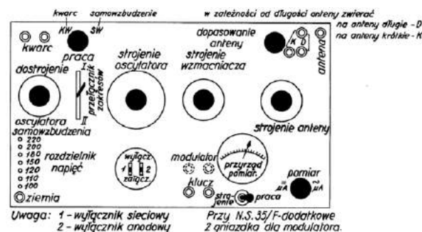
Rys. 5. Szkic płyty czołowej nadainika NS35
