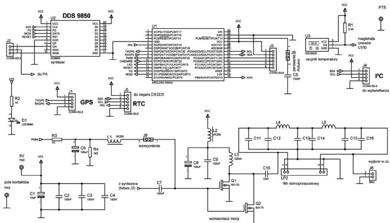
Rys. 3. Schemat ideowy nadajnika F4GOH, wzmacniacza mocy można użyć także w innych projektach. Charakterystyka filtra piątego rzędu opada 30 dB na oktawę
