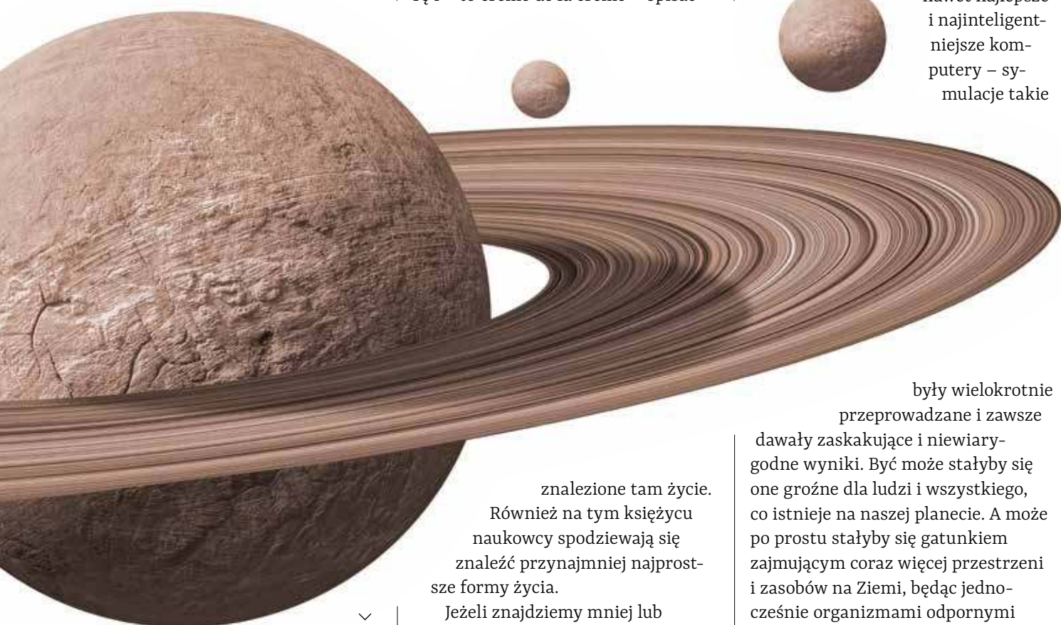
Model Saturna z jego księżycami
