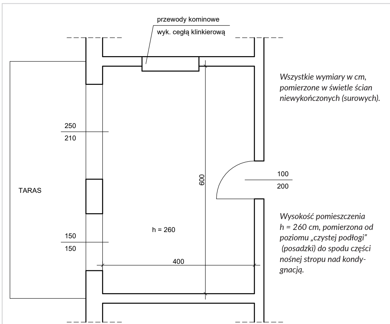
Rzut tynkowanego pomieszczenia – szkic pomocniczy do przedmiaru
