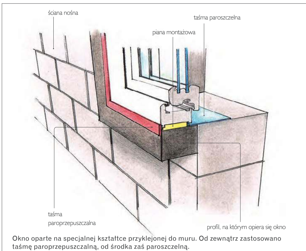
Tylko wysunięcie okien poza lico muru, w warstwę ocieplenia, zastruguje na miano ciepłego montażu. VEKA
