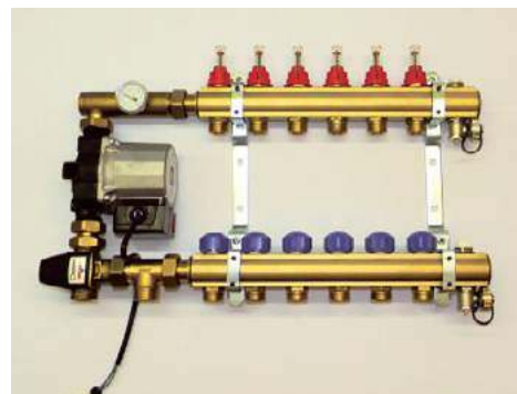
ⓘ Aby połączyć ogrzewaną podłogę z grzejnikami ściennymi, konieczne jest zamontowanie układu mieszającego, który obniży temperaturę wody dopływającej do podłogówki. KISAN
