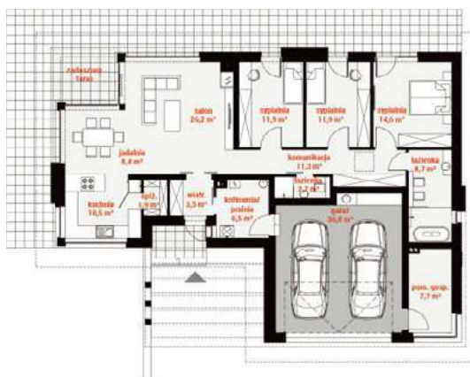
RZUT PARTERU
