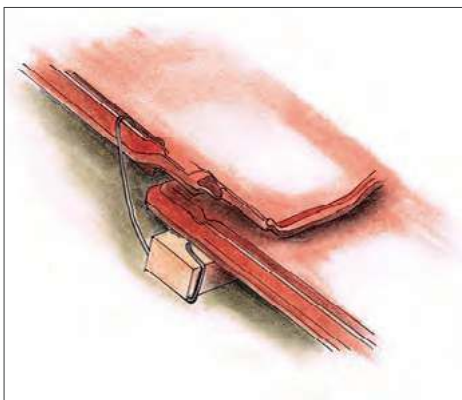
🔧 Mocowanie dachówki za pomocą klamry.
