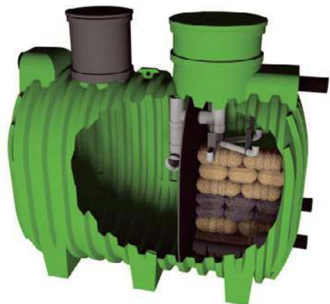
❗ Zbiornik biologicznej oczyszczalni ścieków zbudowany z osadnika wstępnego – wyposażonego w filtr na wylocie, zabezpieczający przed przedostawaniem się części stałych oraz w reaktor ze złożem biofiltracyjnym.
