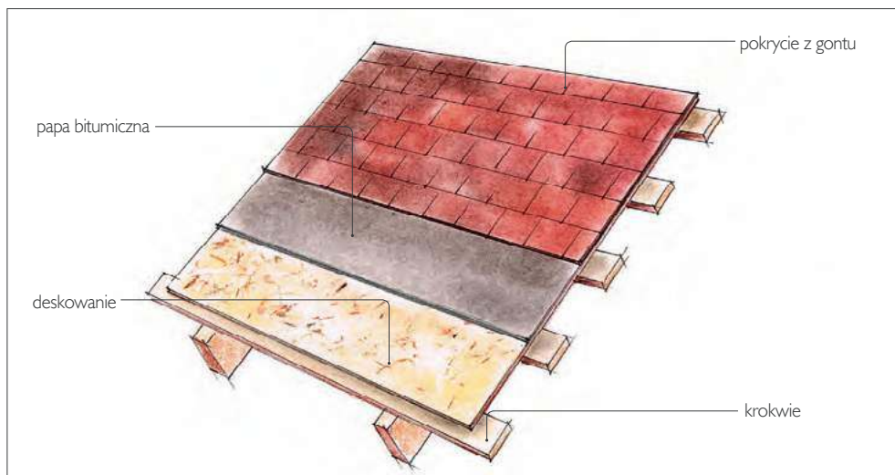
1 Dach pokryty gontem bitumicznym.
