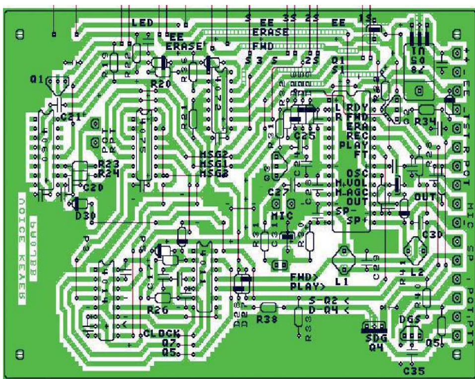
Rys. 6. Główna płytką drukowaną Voice Keyer
