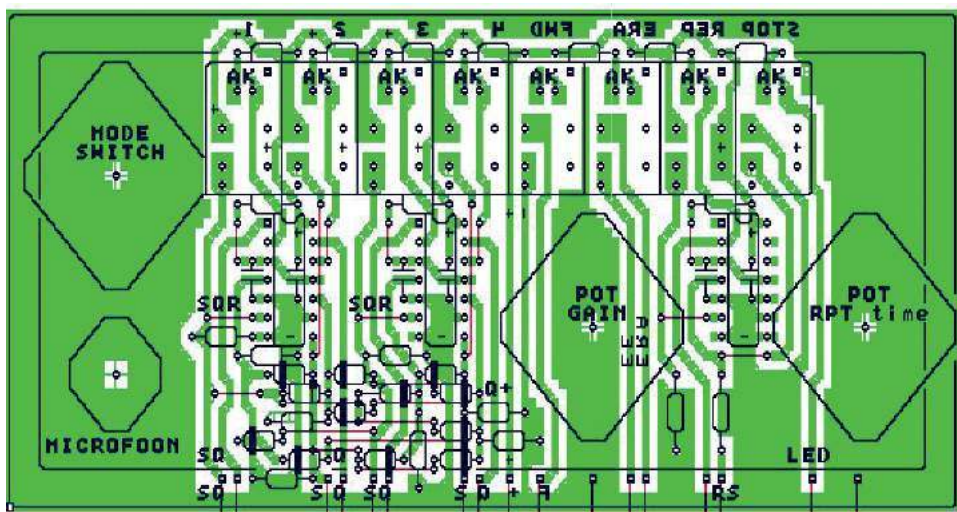
Rys. 7. Płytką czołową Voice Keyer
