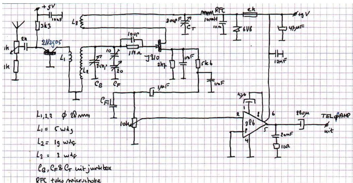
Rys. 4. Schemat odbiornika reakcyjnego
