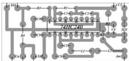
Rys. 3. Rozmieszczenie elementów na płycie nadajnika CW
