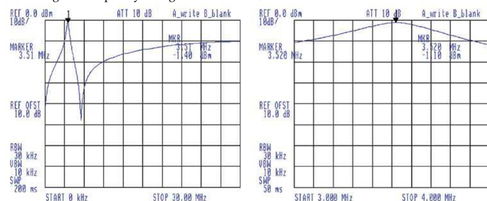
Rys. 5. Charakterystyka filtra pasmowo-przepustowego RX
