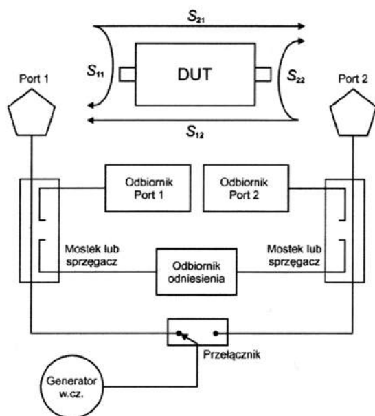
Rys. 2. Uproszczony schemat blokowy analizatora sieci
