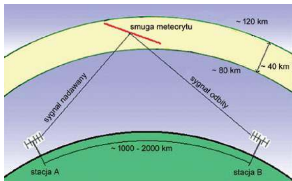
Rys. 1. Łączność za pośrednictwem odbić od zjonizowanych smug meteorów (MS)
