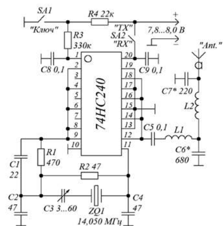
Rys. 2. Schemat nadajnika CW na układzie 74HC240
