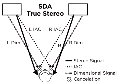
Rys. 2. Para głośników z systemem SDA: linie ciągłe: sygnały pożądane, linie kropkowane: sygnały powodujące przesłuch, linie szare: sygnały różnicowe, znikające z sygnałami powodującymi przesłuch.
