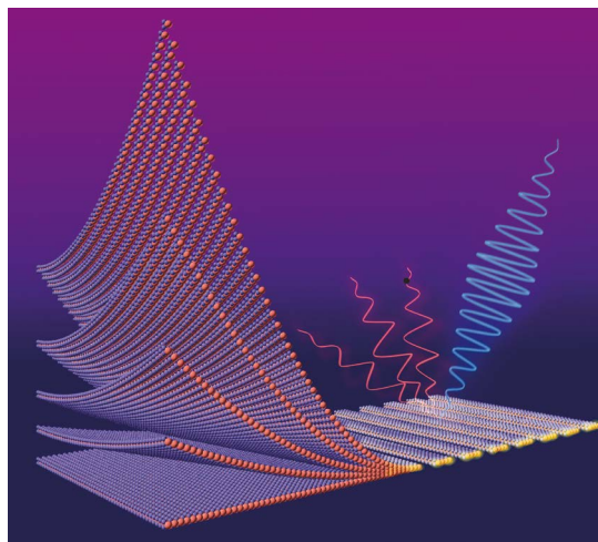
Siatka MoSe 2 . Siatka podfalowa z warstwowego diselenku molibdenu – wizja artystyczna. Czerwone kulki symbolizują atomy molibdenu, niebieskie – selenu. Światło zostaje uwięzione w siatce, co wzmacnia generację światła o potrojonej częstotliwości.
