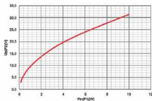
Rys. 6. Wykres wartości szczytowej napięcia w funkcji mocy oddawanej do obciążenia
