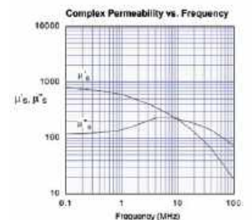
Rys. 2. Materiał 43 firmy Amidon – parametry \mu' oraz \mu''
