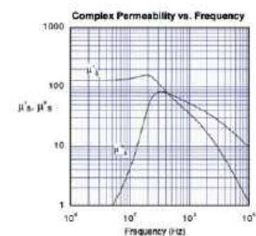
Rys. 3. Charakterystyki \mu' , \mu'' materiałów (od góry: 31, 43 i 61)
