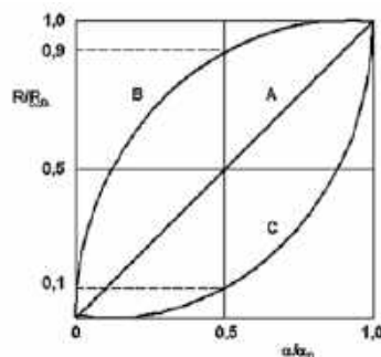
Rys. 2. Oznaczenia charakterystyki potencjometrów polskiej produkcji
