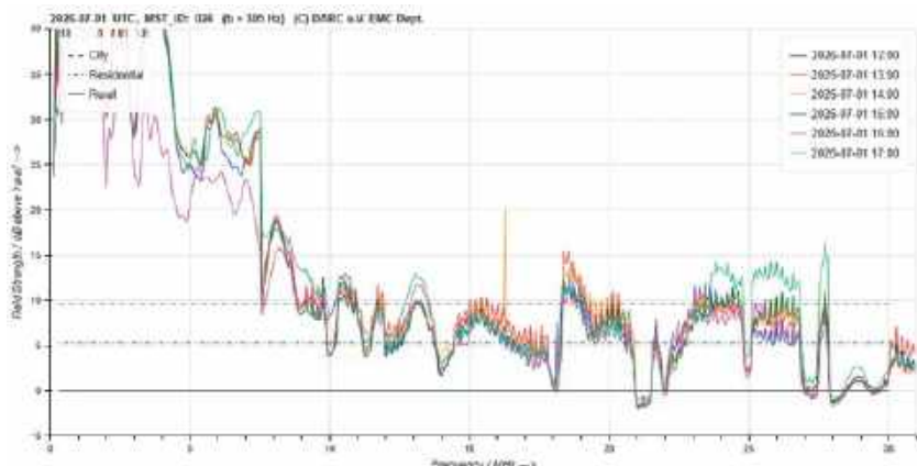
WYKRESY WIDMOWE DLA 6 GODZIN ENAMS
