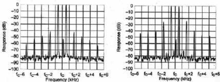
Rys. 2. Po prawej stronie widmo sygnału z włączoną korekcją w paśmie 14 MHz. Szerokość widma wynosi ±6 kHz wokół nośnej, poziomem odniesienia jest 0 dBc, podziałki skali pionowej 10 dB. Po prawej stronie widmo w paśmie 14 MHz przy użyciu tej samej radiostacji IC-7760, ale z wyłączoną korekcją
