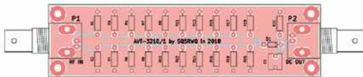
Rys. 5. Rozmieszczenie elementów na płytce drukowanej AVT 3210
