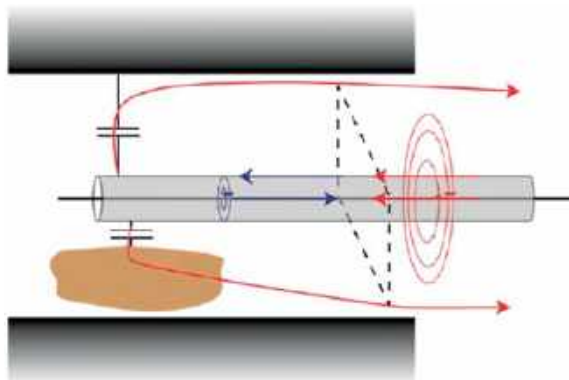
Rys. 1. Powstawanie i rozptyw prądu common-mode (czerwone strzałki) oraz prądu różnicowego (niebieskie strzałki).
