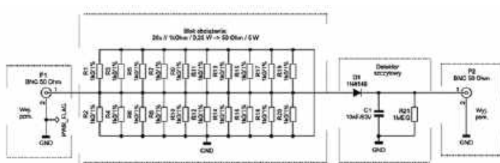
Rys. 4. Schemat sztucznego obciążenia 50 Ω/5 W
