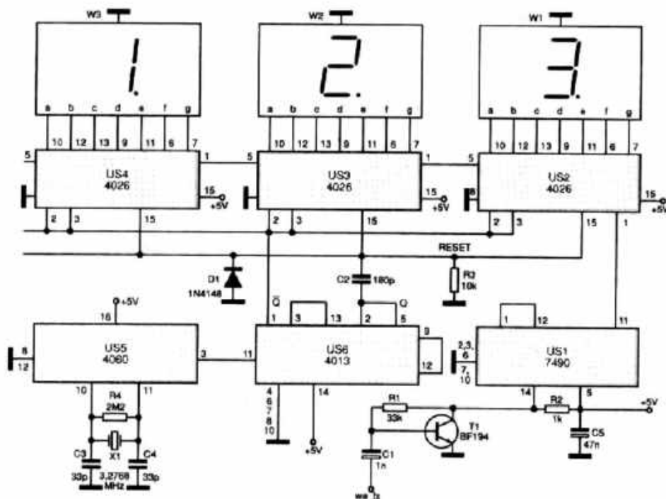
Rys. 3. Schemat skali częstotliwości AVT135
