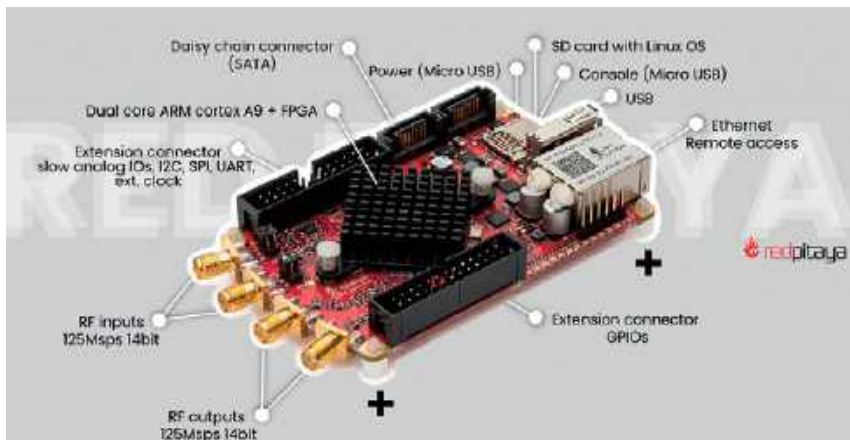
SERCE ODBIORNIKA ENAMS
