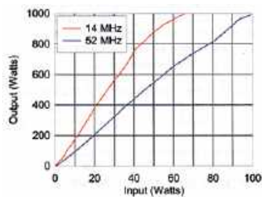
Rys. 1. Zależność mocy wyjściowej od wejściowej w paśmie 14 MHz (linia czerwona) i 50 MHz (linia niebieska)
