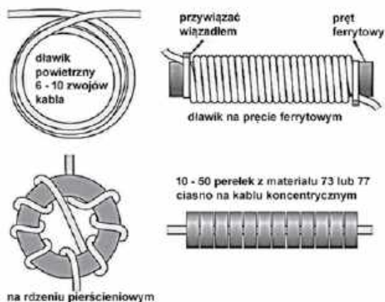
Rys. 1. Różne konstrukcje dławików antenowych
