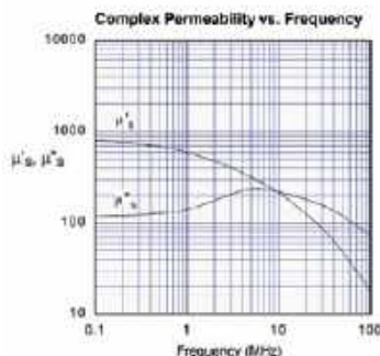
Rys. 2. Materiał 43 firmy Amidon – parametry \mu' oraz \mu''
