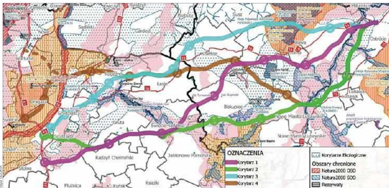
Cztery korytarze przebiegu S5 z Grudziądza do Ostródy
