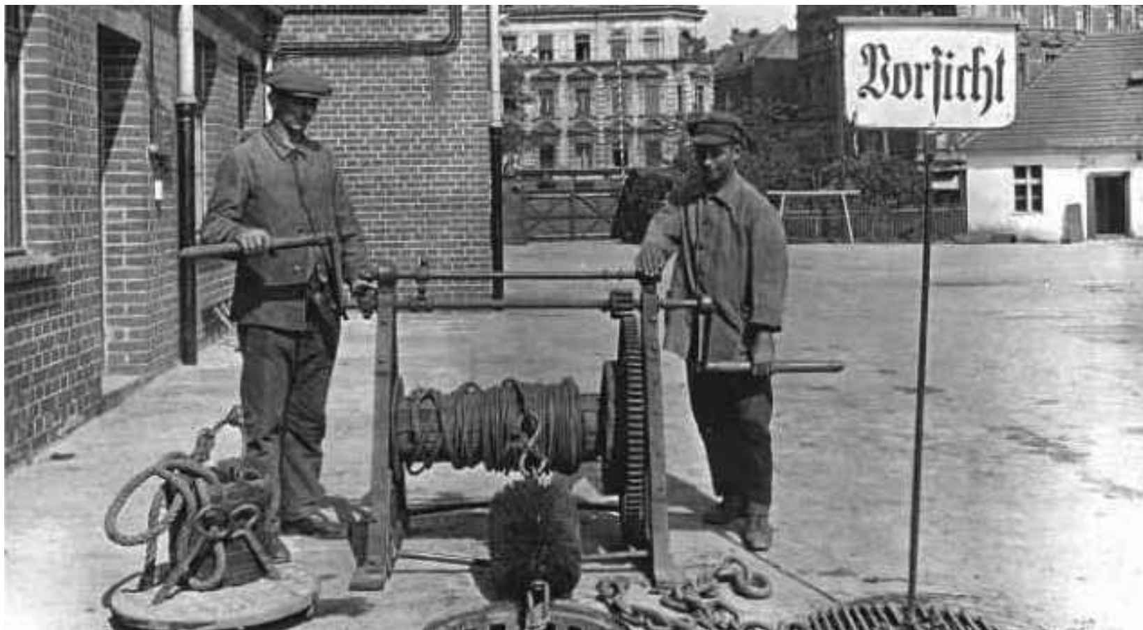
Ekipa sieci kanalizacyjnej przy pracy
