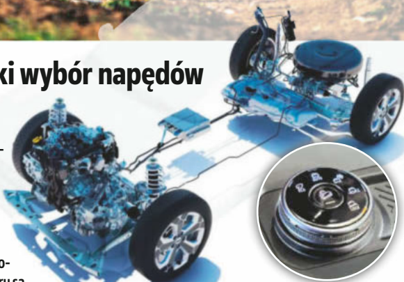
Wyjątkowe rozwiązanie: dwupaliwowy układ MHEV z napędem na 4 koła.
