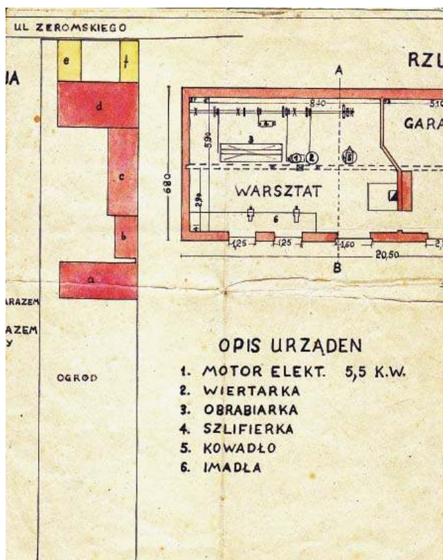
Plan sytuacyjny posesji (pp. Rexin) Michalskich przy ul. Żeromskiego nr 10. (6a), a) dom, b) garaż, c) kuźnia, d) szopa przed domem, e i f) bud. gospodarcze. Nidzica, 12 VII 1948 r. (Zbiory autora)
